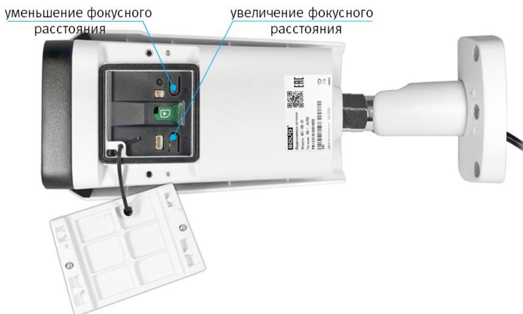
Рисунок 5.3 – Настройка фокусного расстояния вручную
