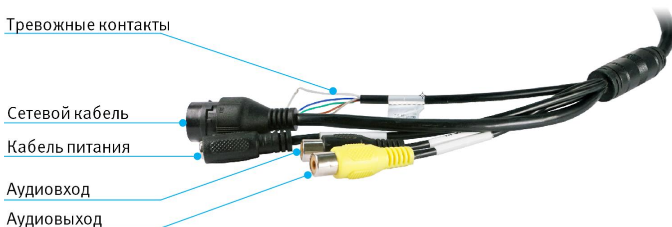
Рисунок 6.1 – Кабель видеокамеры
