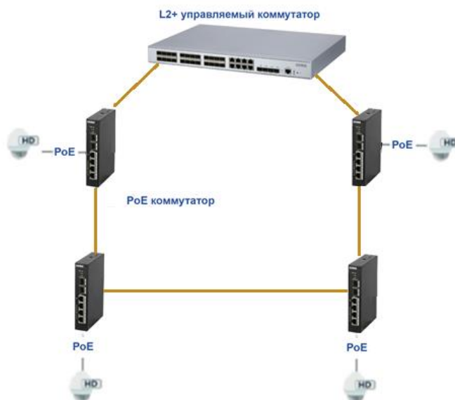
Рисунок 1.2 Кольцевое соединение
