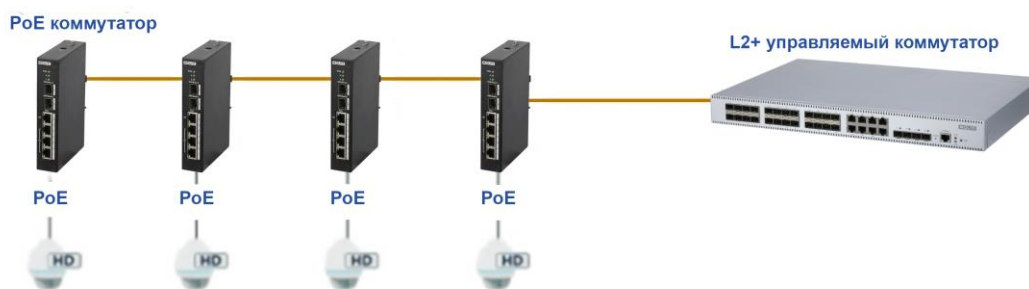
Рисунок 1.1 Каскадное соединение
