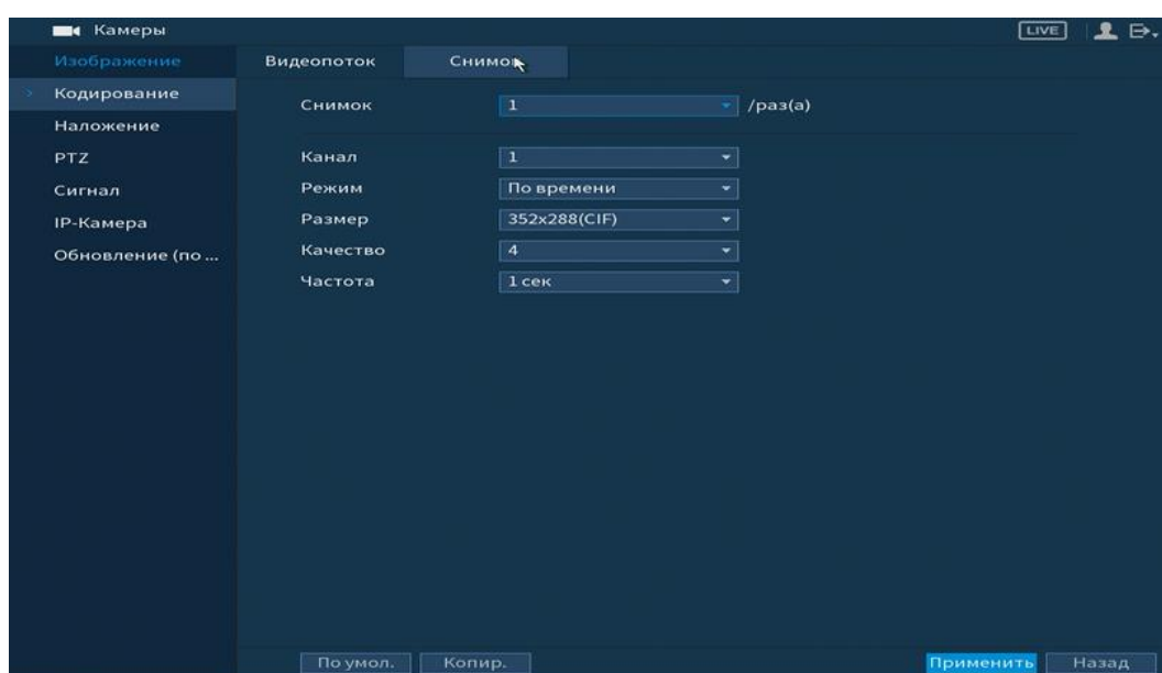
Рисунок 6.74 Настройка снимка
