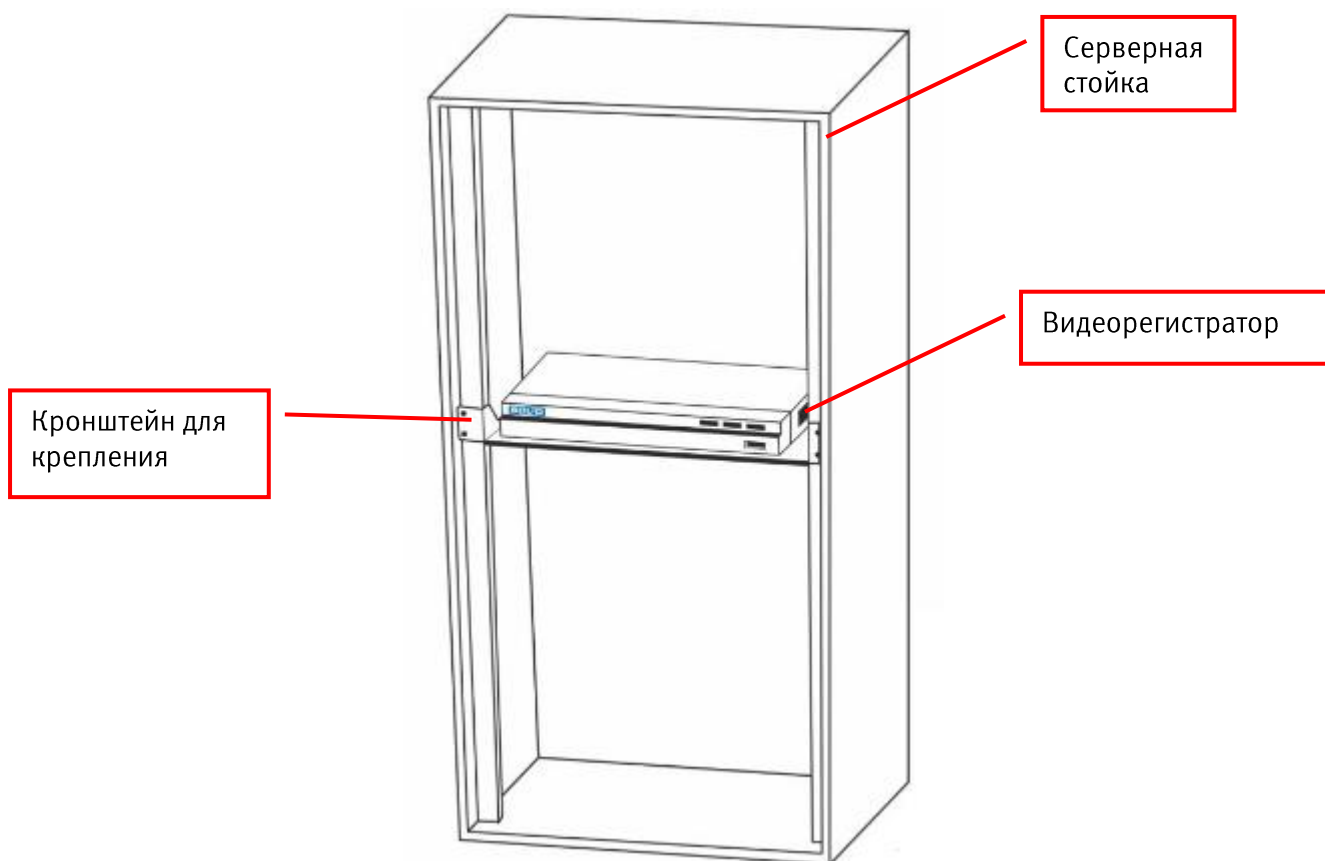
Рисунок 3.12 Монтаж видеорегистратора в 19"- стойку с помощью кронштейна
