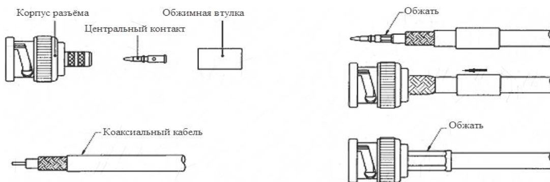
Рисунок 3.10 Схема обжима BNC
