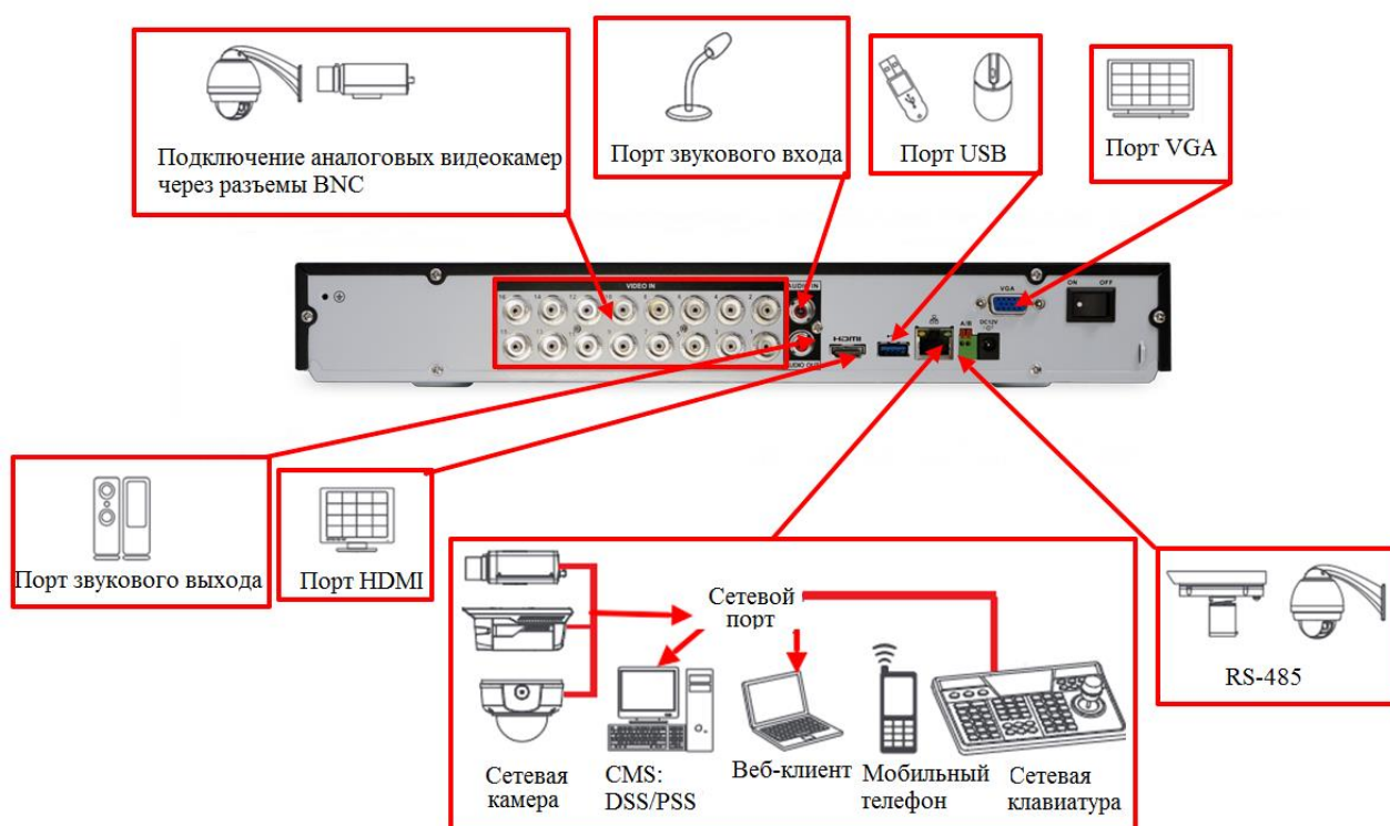
Рисунок 3.2 Внешний вид задней панели
