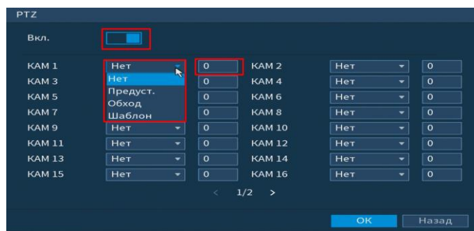
Рисунок 6.46 Настройка предустановки
