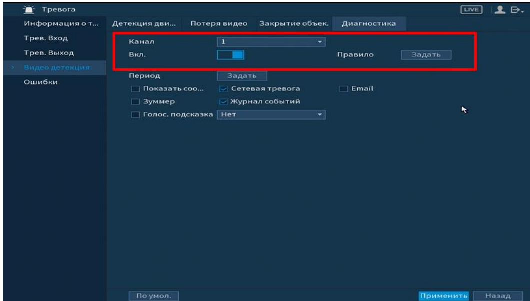
Рисунок 6.32 Диагностика
