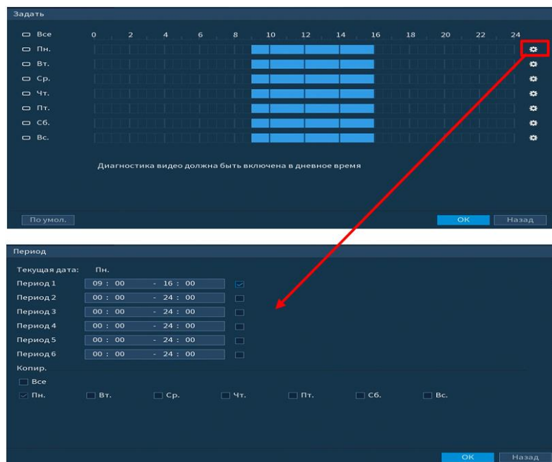
Рисунок 6.34 Настройка расписания
