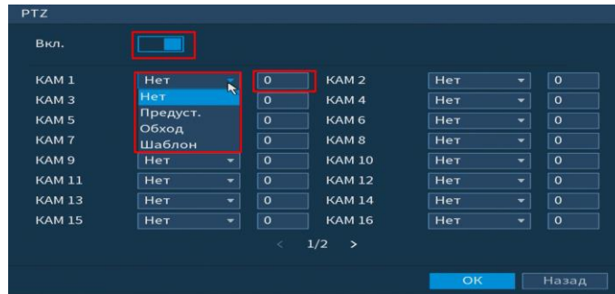
Рисунок 6.16 Настройка предустановки
