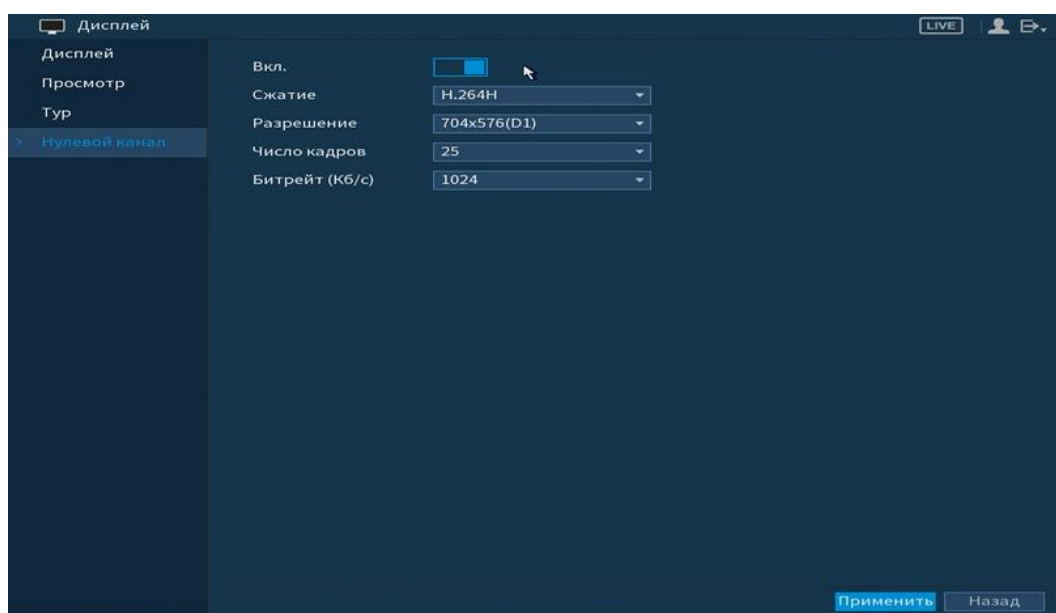
Рисунок 6.69 Интерфейс настройки
