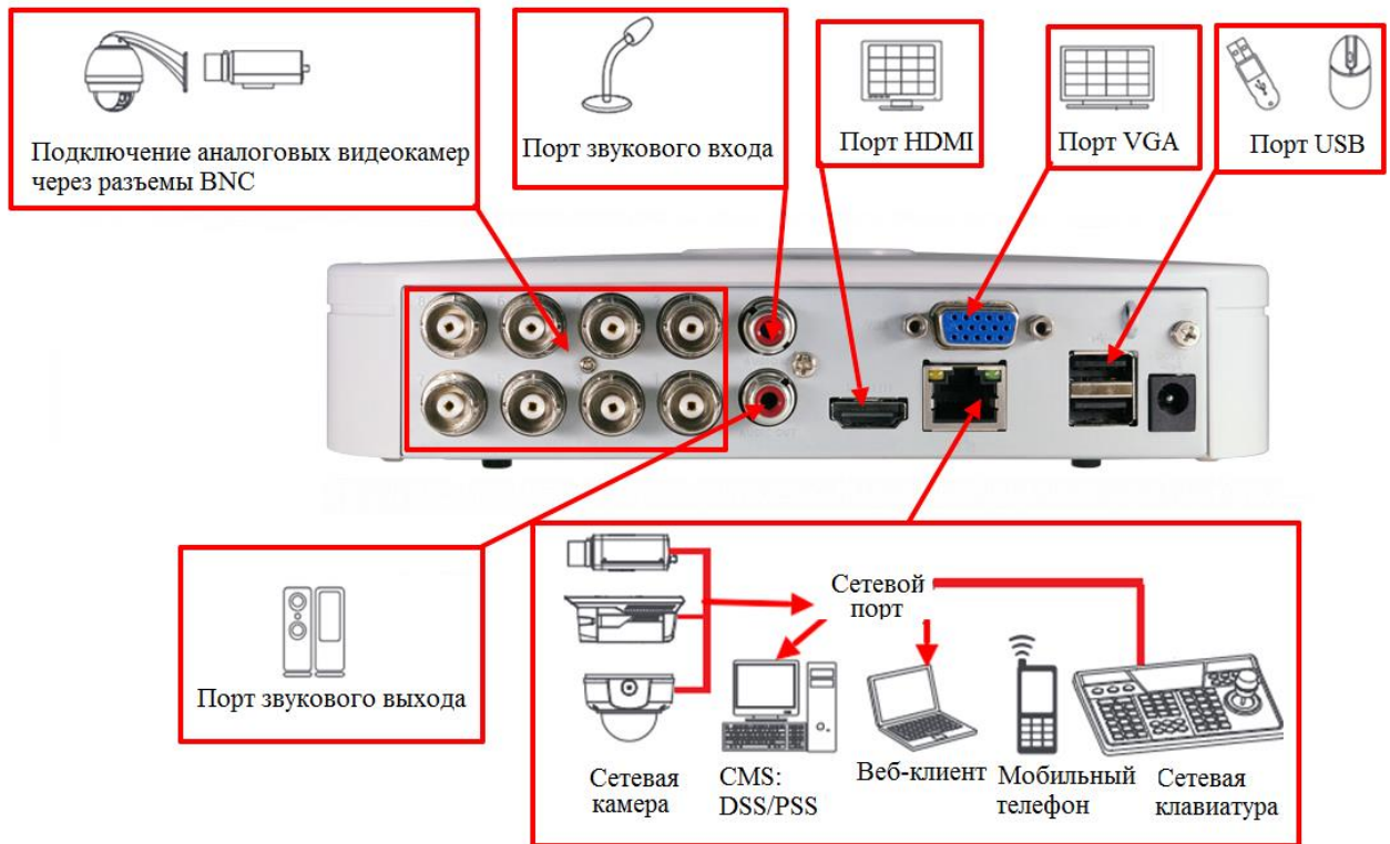
Рисунок 3.2 Внешний вид задней панели
