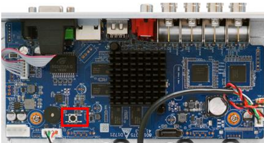
Рисунок 6.96 Возможный пример нахождения кнопки сброса
