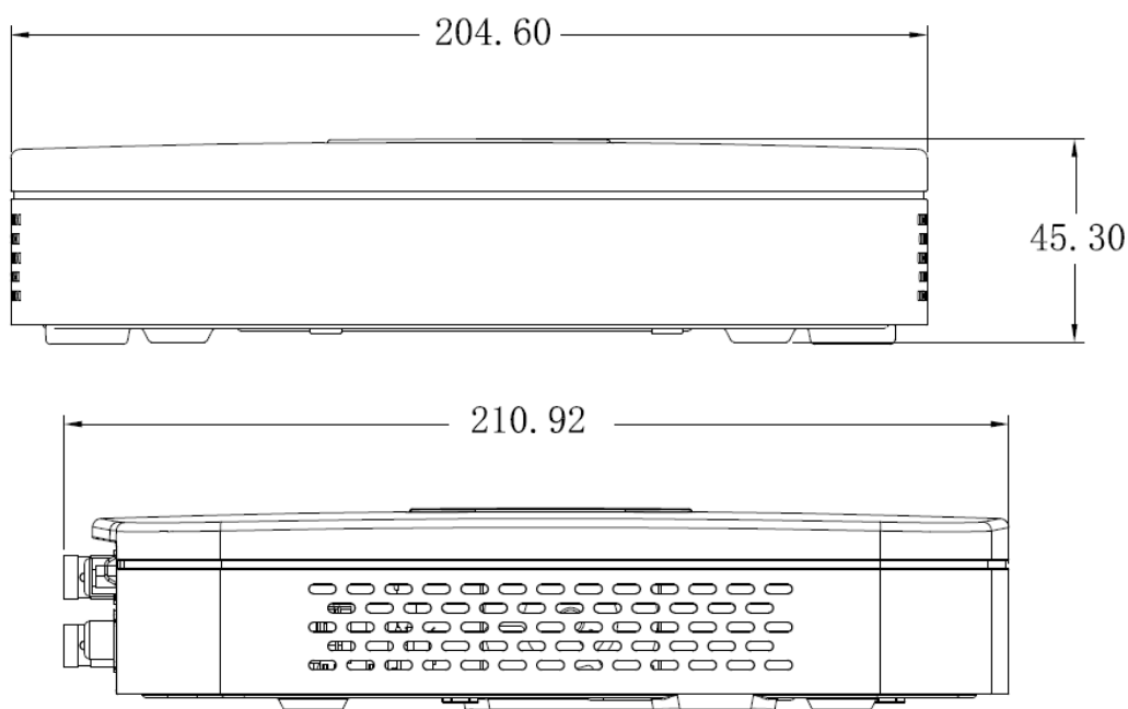
Рисунок 3.9 Габаритные размеры видеорегистратора
