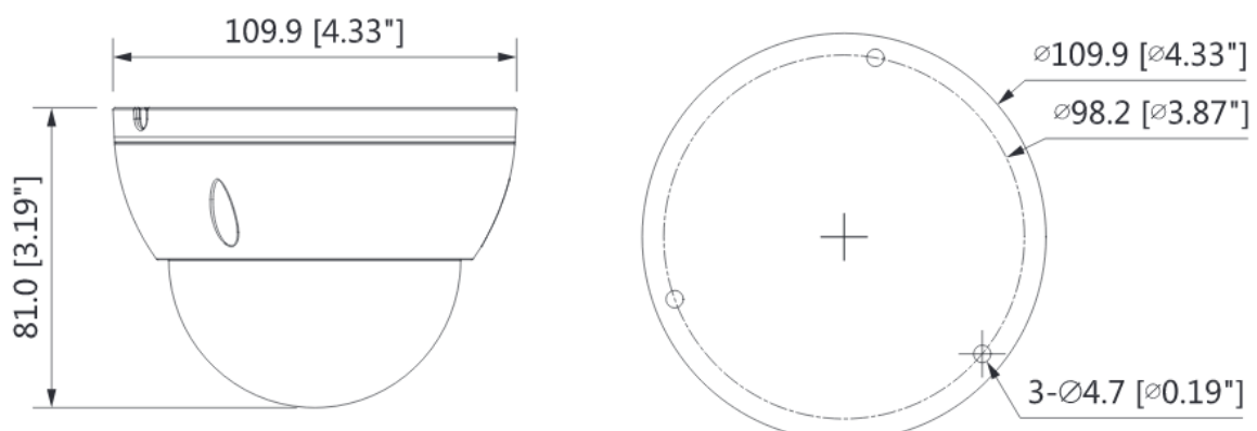
Рисунок 5.1 — Габаритные размеры видеокамеры
