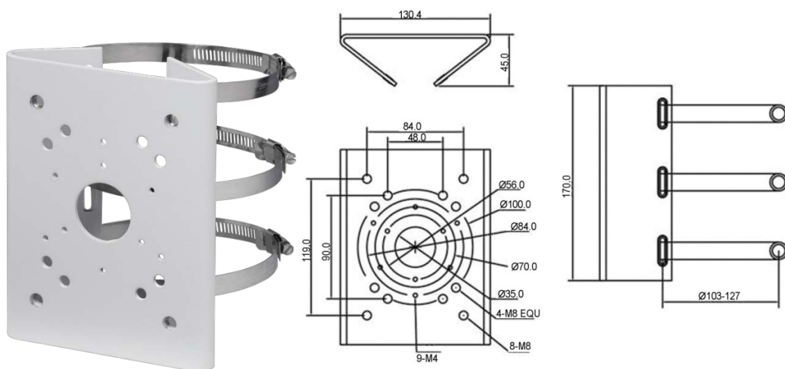
Рисунок 5.7 — Столбовой кронштейн BR-103
