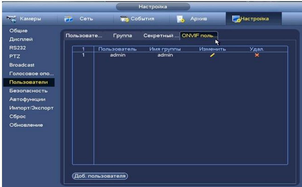
Рисунок 8.197 Настройка ONVIF.
