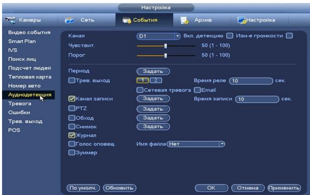
Рисунок 8.122 Настройка аудиодетекция.
