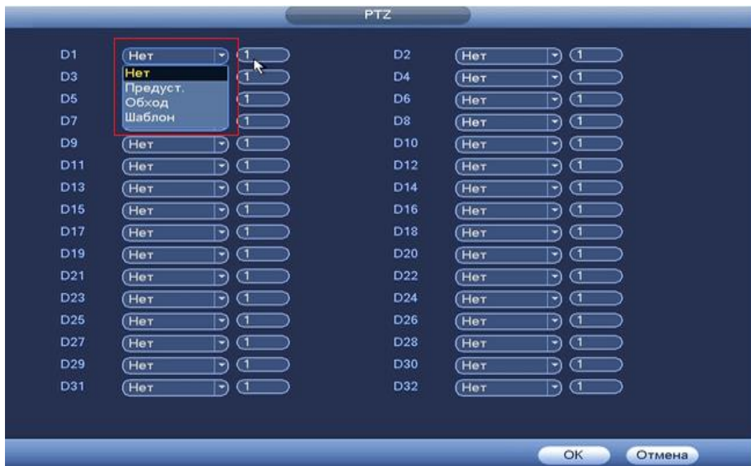
Рисунок 8.118 Установка предустановок.
