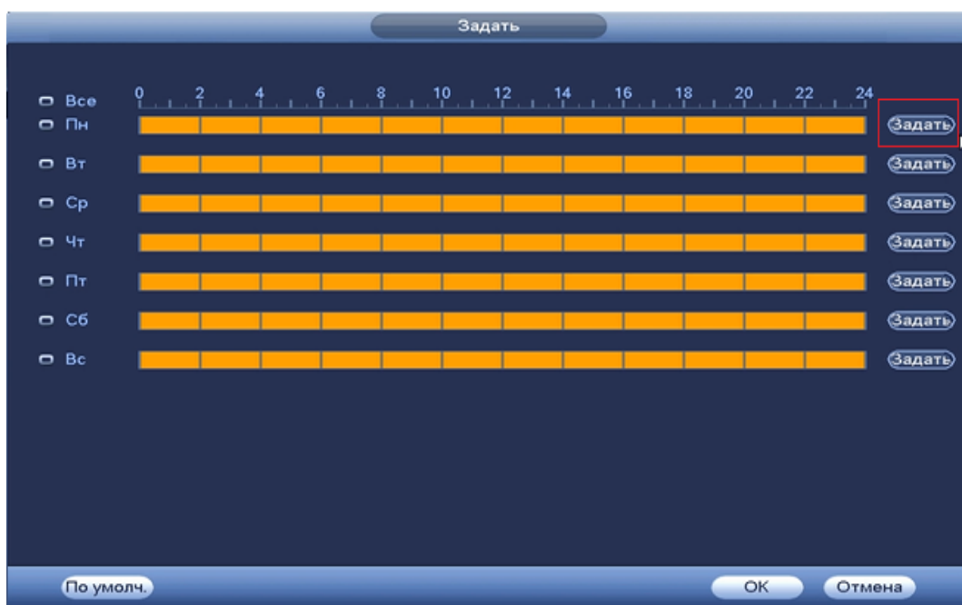
Рисунок 8.139 Настройка расписания.
