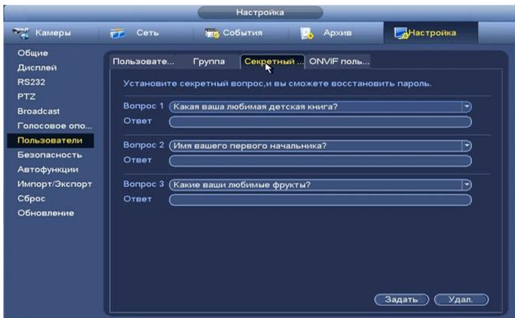
Рисунок 8.196 Интерфейс настройки
