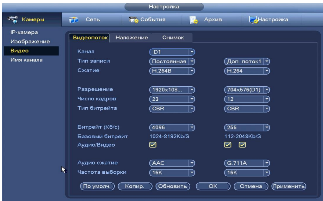
Рисунок 8.44 Интерфейс настройки видеопотоков.
