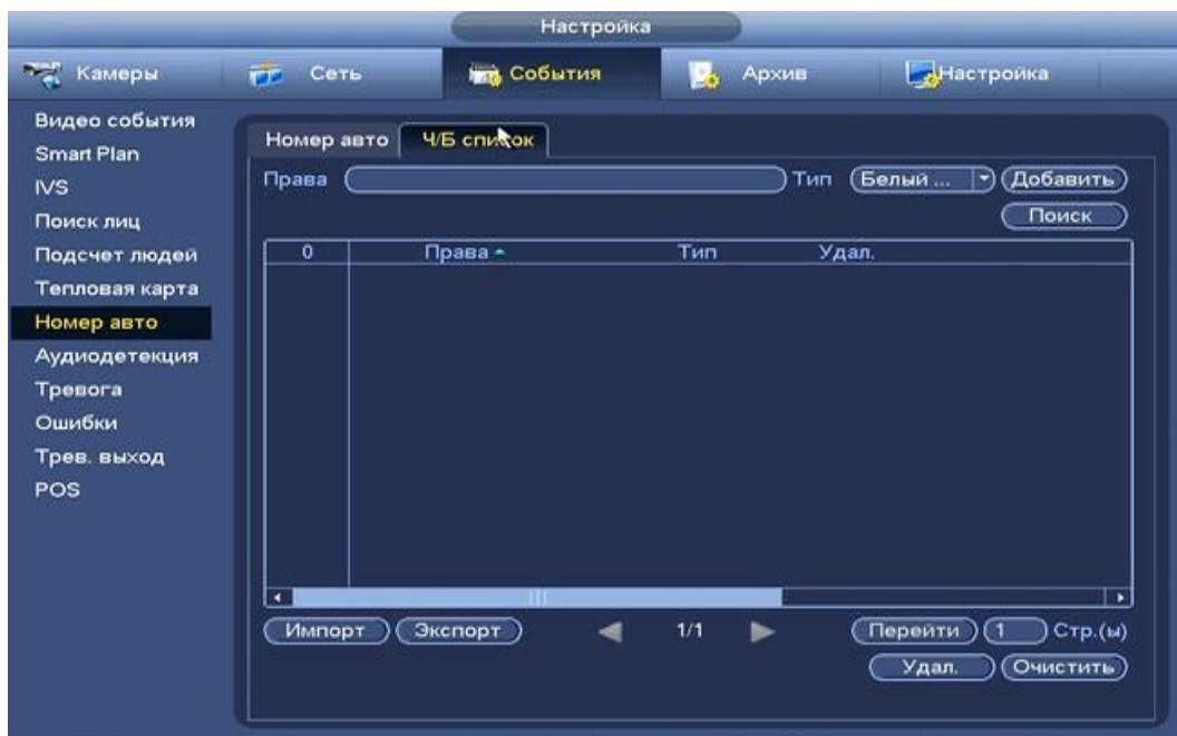
Рисунок 8.121 Ч/Б список
