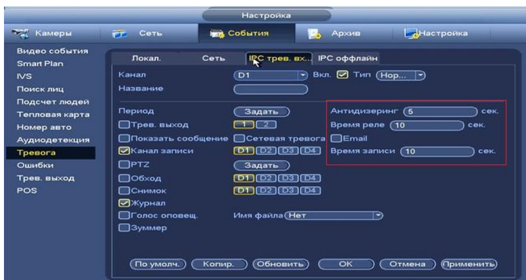
Рисунок 8.142 Установка настроек.
