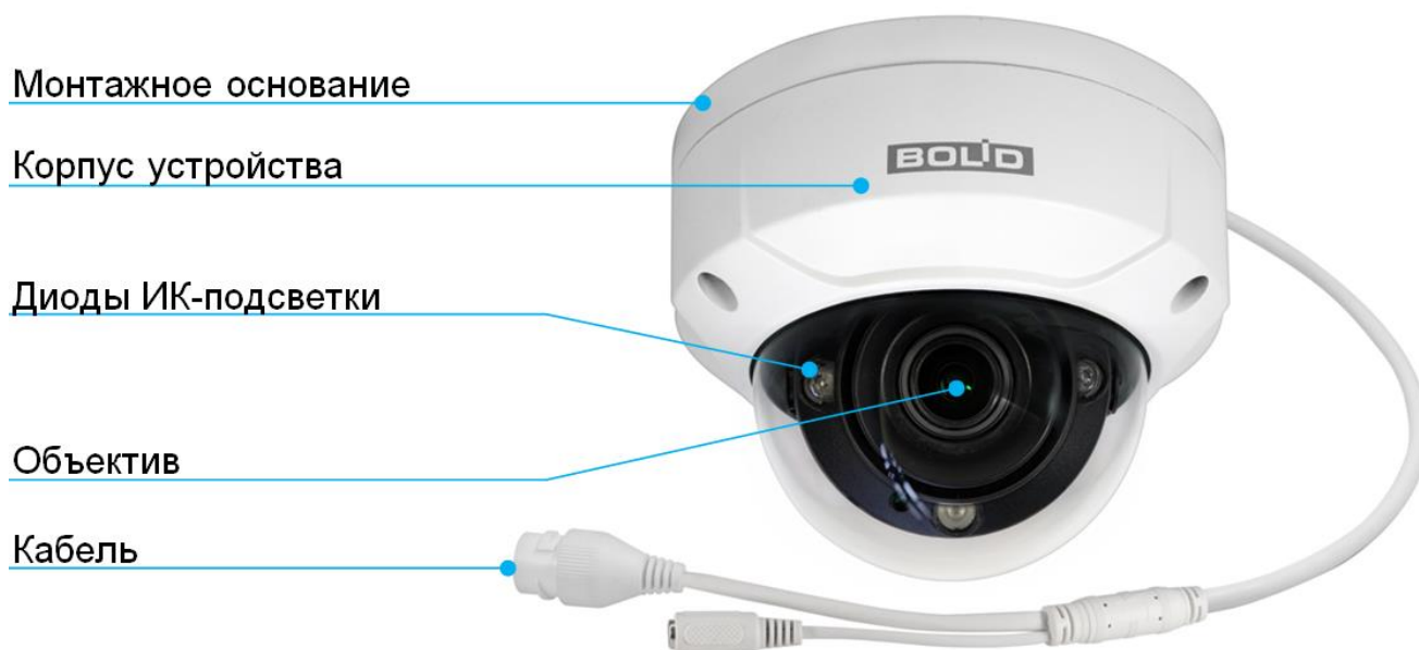
Рисунок 4.1 - Внешний вид и основные элементы видеокамеры
