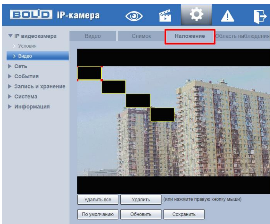
Рисунок 7.41 – Вкладка «Наложение»
