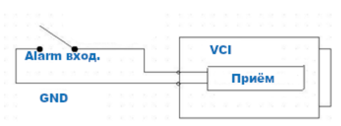
Рисунок 6.5 — Схема подключения тревожного входа
