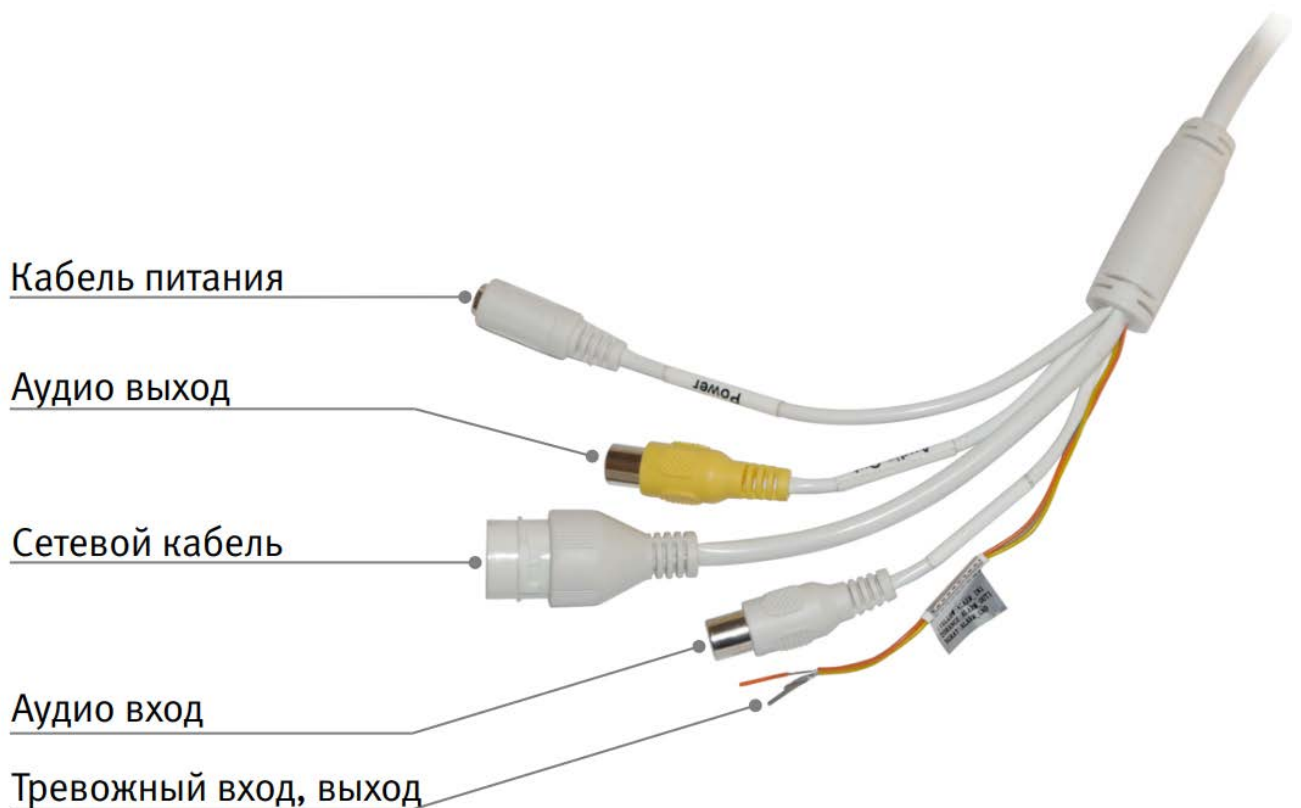
Рисунок 6.1 — Кабель видеокamеры
