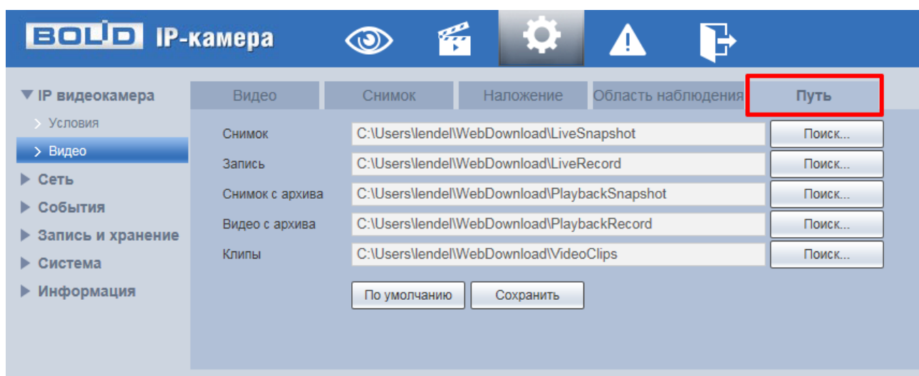
Рисунок 7.48 – Вкладка «Путь»
