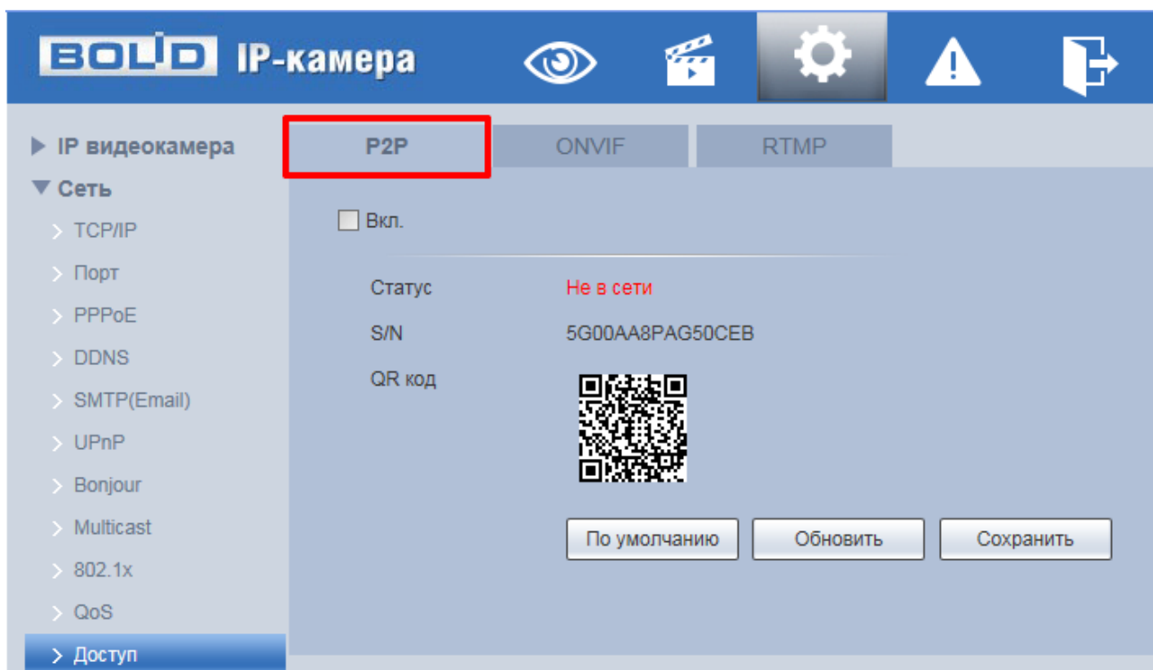
Рисунок 7.65 - Вкладка «P2P»
