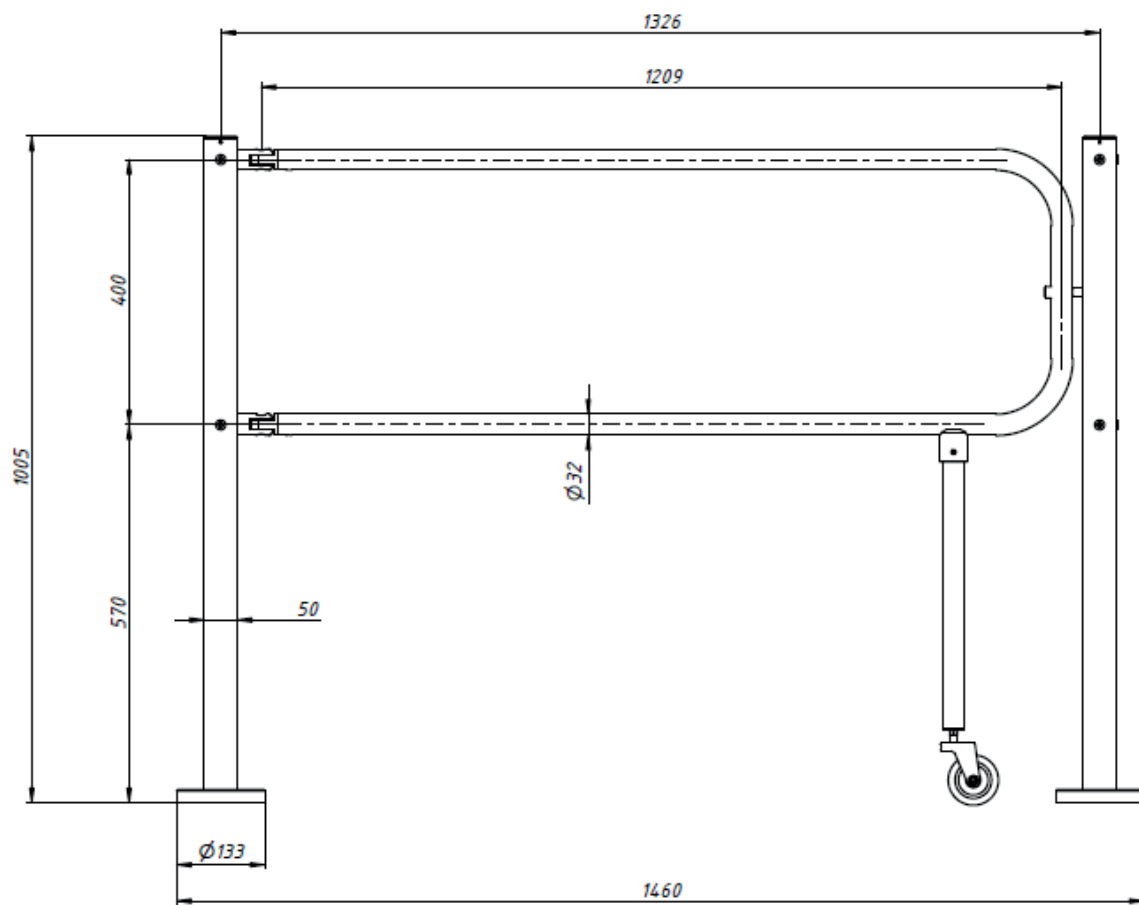
Рисунок 4.1 Габаритные размеры секции Антипаника «RTA-011»
