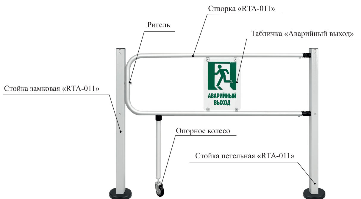
Рисунок 6.1 Состав секции Антипаника «RTA-011»
