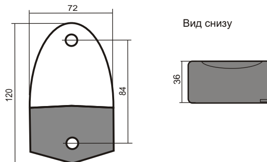
Рис.1. Габаритные и установочные размеры оповещателя
