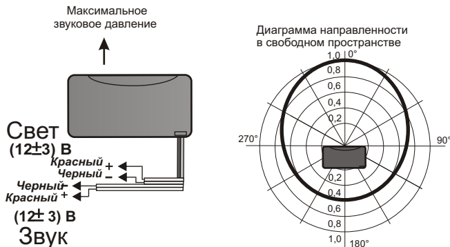
Рис.2 Схема подключения и диаграмма направленности звука оповещателя.
