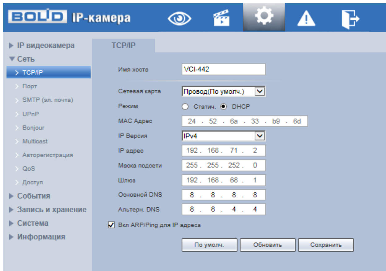
Рисунок 7.50 — Пункт меню «Сеть»
