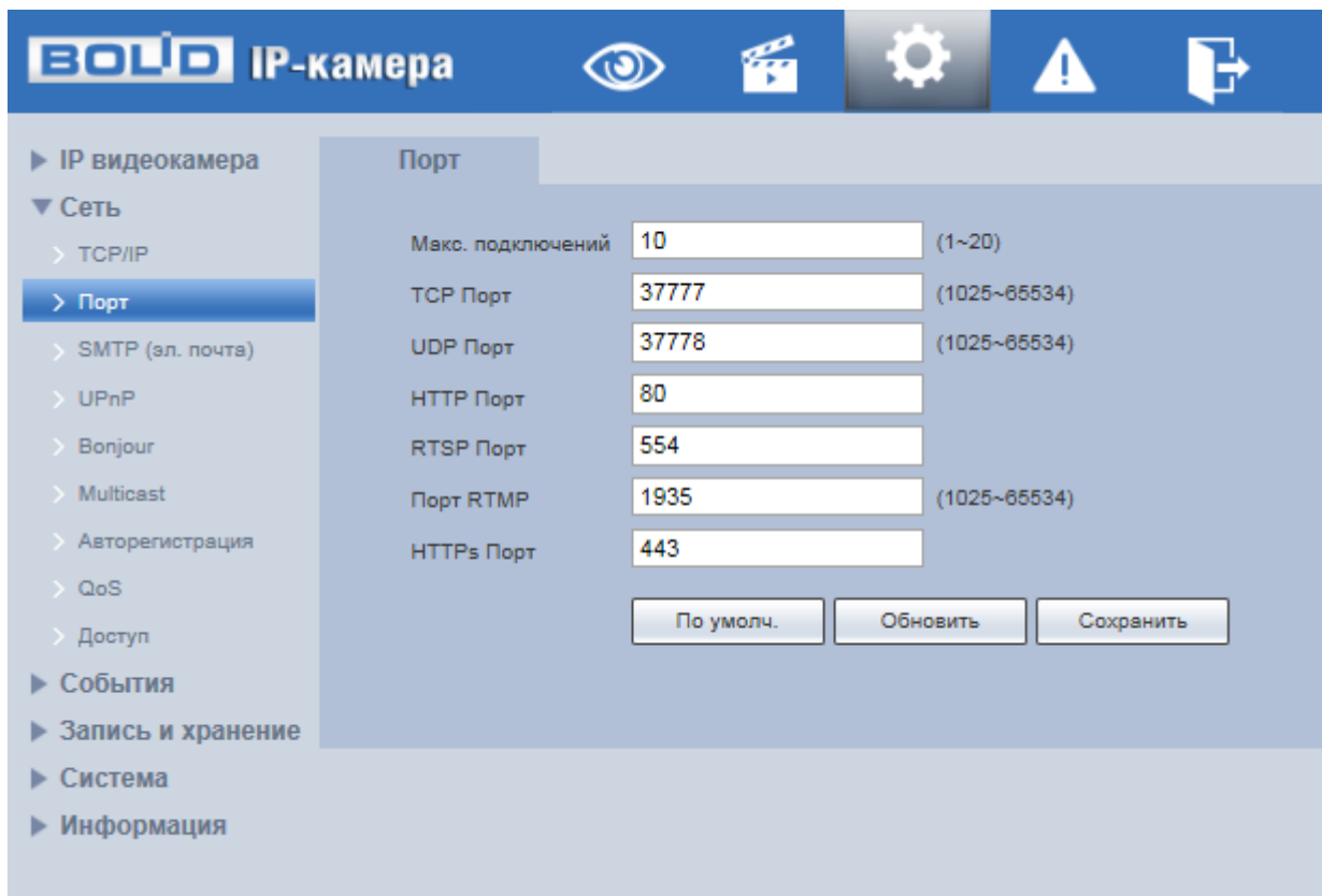
Рисунок 7.53 — Подпункт меню «Порт»
