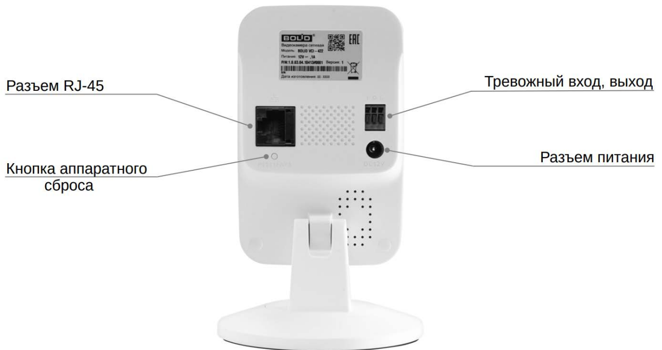
Рисунок 6.1 — Разъемы видеокамеры
