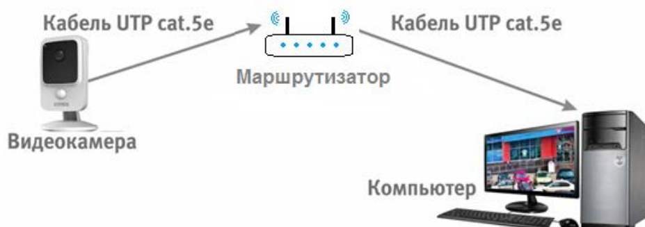
Рисунок 6.3 — Схема подключения видеочамеры к компьютеру по Wi-Fi
