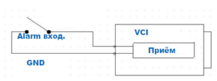
Рисунок 6.6 — Схема подключения тревожного входа
