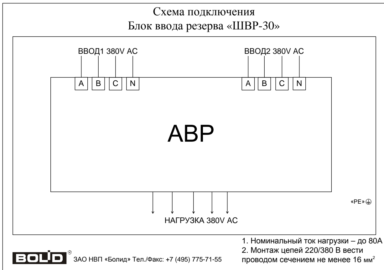
Рисунок 5. Схема внешних соединений ШВР-30.
