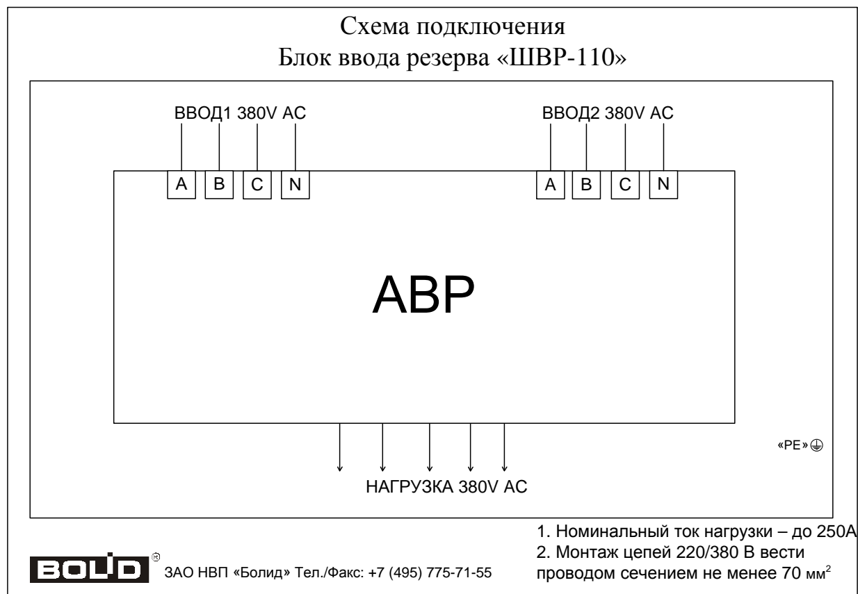
Рисунок 6. Схема внешних соединений ШВР-110.
