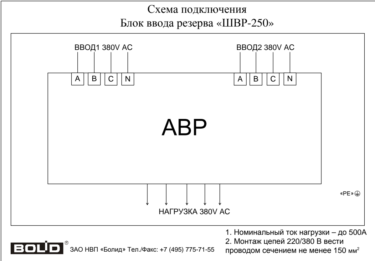
Рисунок 7. Схема внешних соединений ШВР-250.
