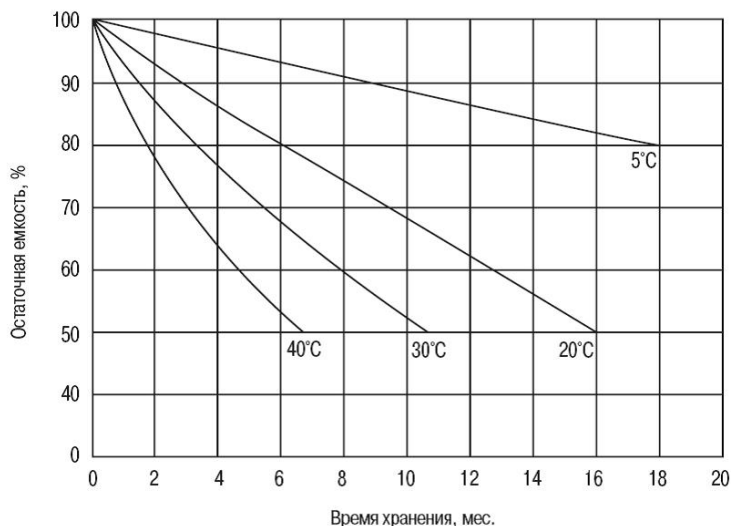
Рис. 9. Зависимость остаточной ёмкости от времени хранения при различных значениях температуры батареи.
