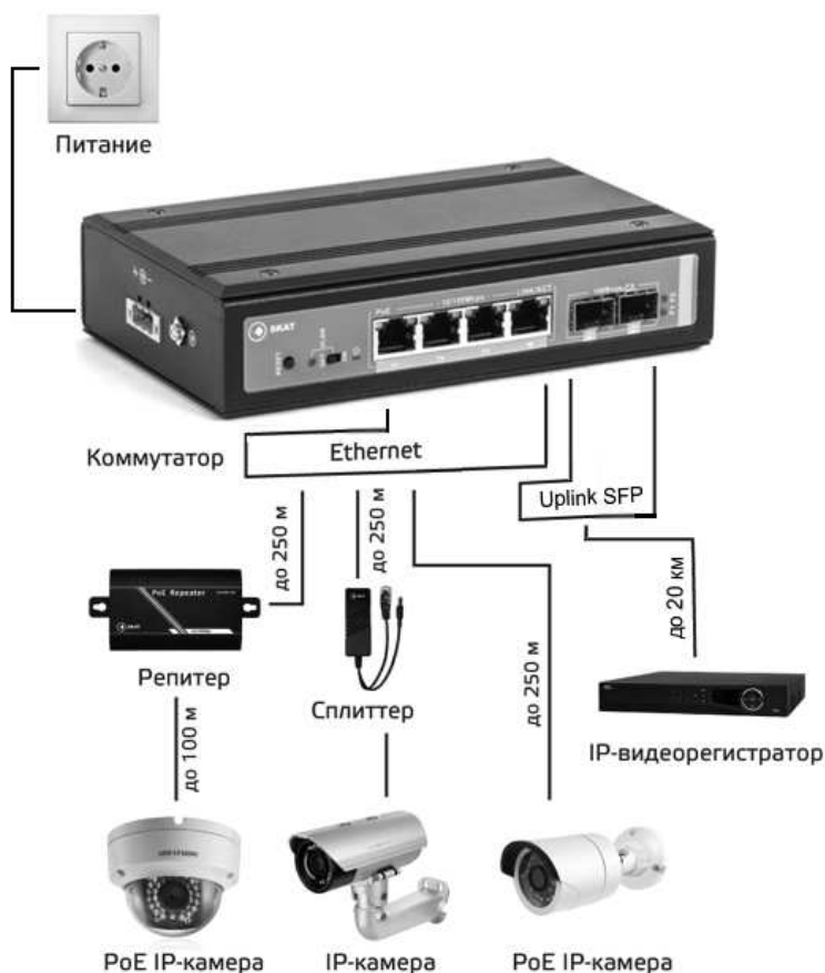
Рисунок 4 – Общая схема подключения устройств к коммутатору
