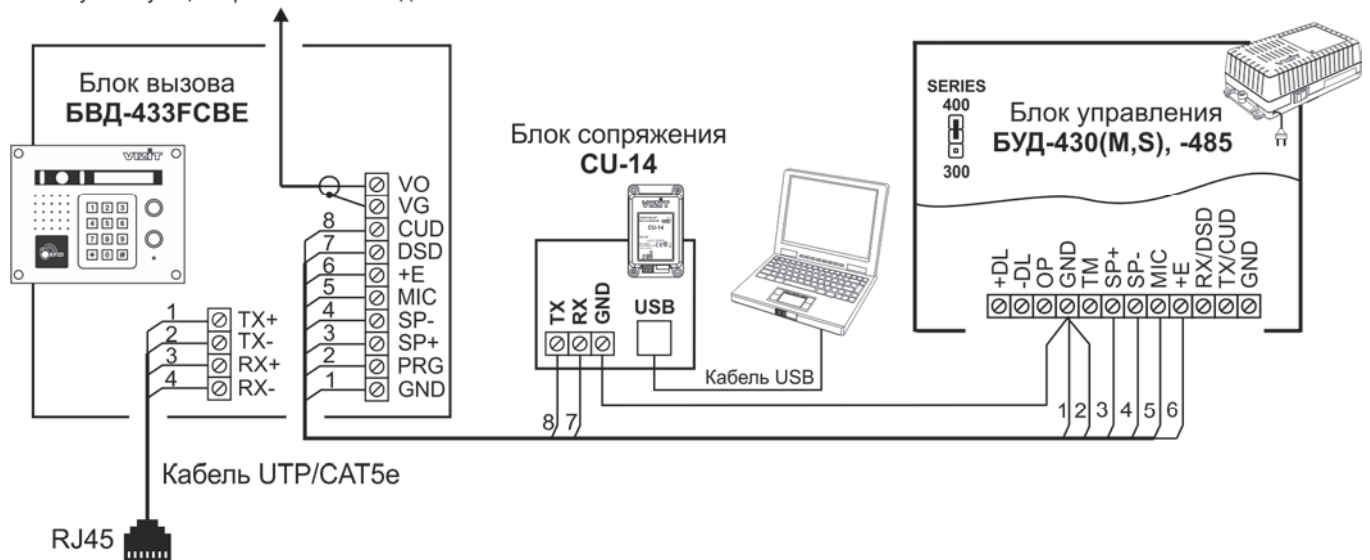
Рисунок 15.1 - Схема соединений блока вызова с блоками управления БУД-430(С, М), -485 и блоком сопряжения CU-14
