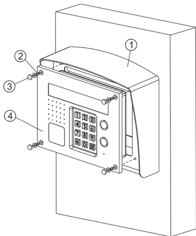
Рисунок 6.3 - Установка блока вызова на монтажный комплект МК-432
