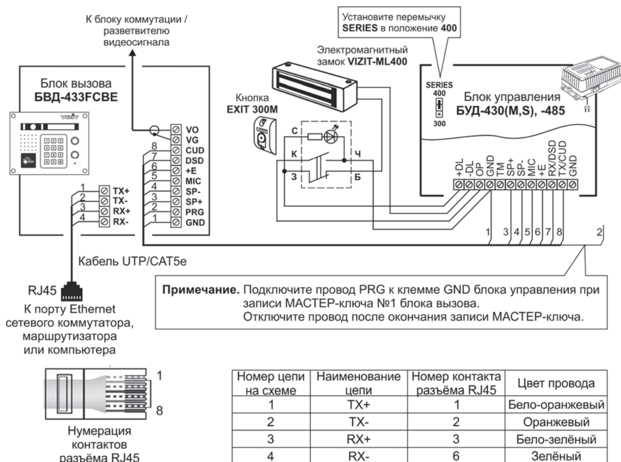
Рисунок 8.1 – Схема соединений блока вызова БВД-433ФСВЕ с блоком управления БУД-430(М, S), -485(М), электромагнитным замком VIZIT-ML400 и кнопкой EXIT 300M
