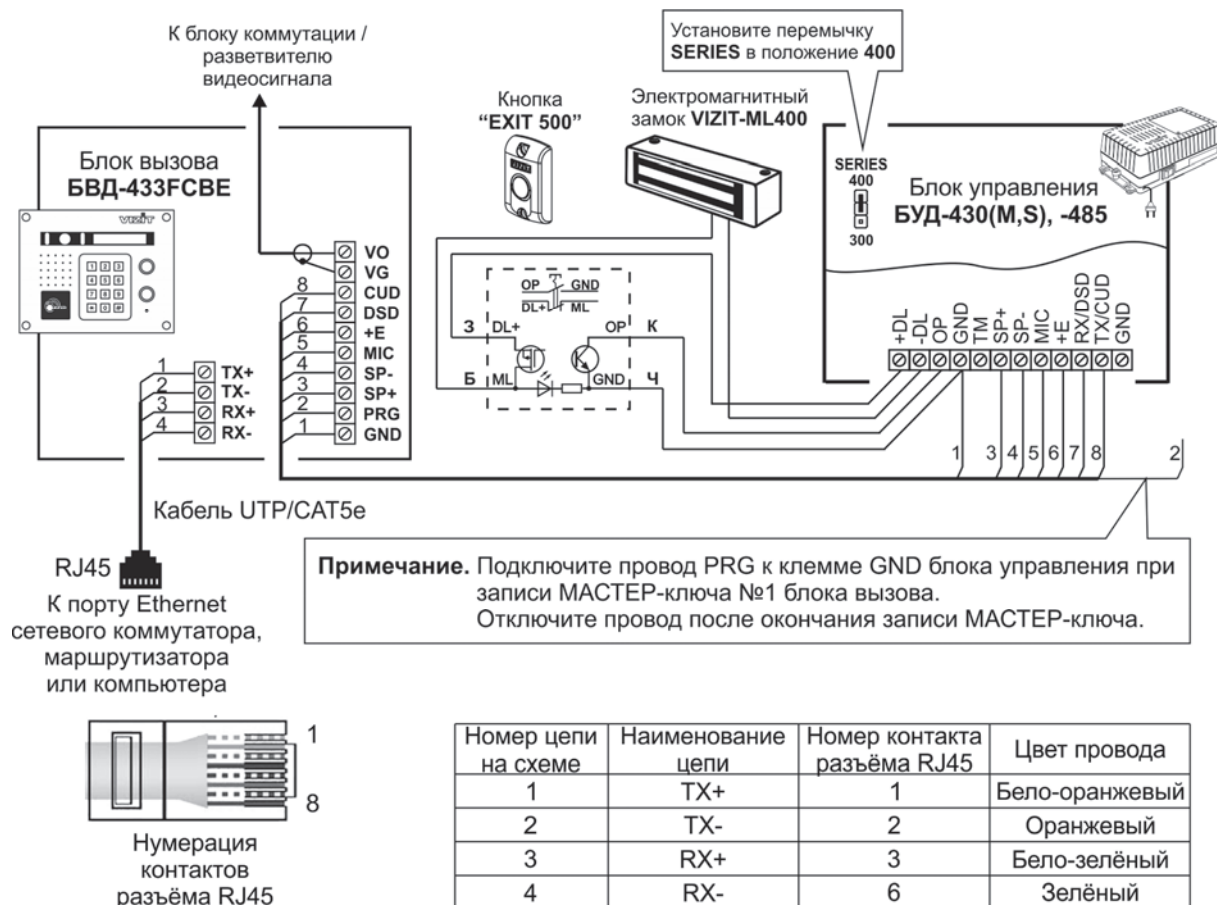
Рисунок 8.2 – Схема соединений блока вызова БВД-433ФСВЕ с блоком управления БУД-430(М, S), -485(М), электромагнитным замком VIZIT-ML400 и кнопкой EXIT 500
