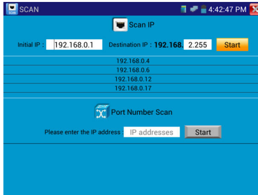
Рис.3.3.6-1 Окно сканирования IP-адресов
