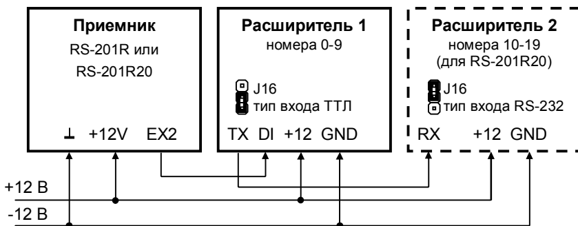
Рис. 3. Подключение расширителя к приёмникам RS-201
