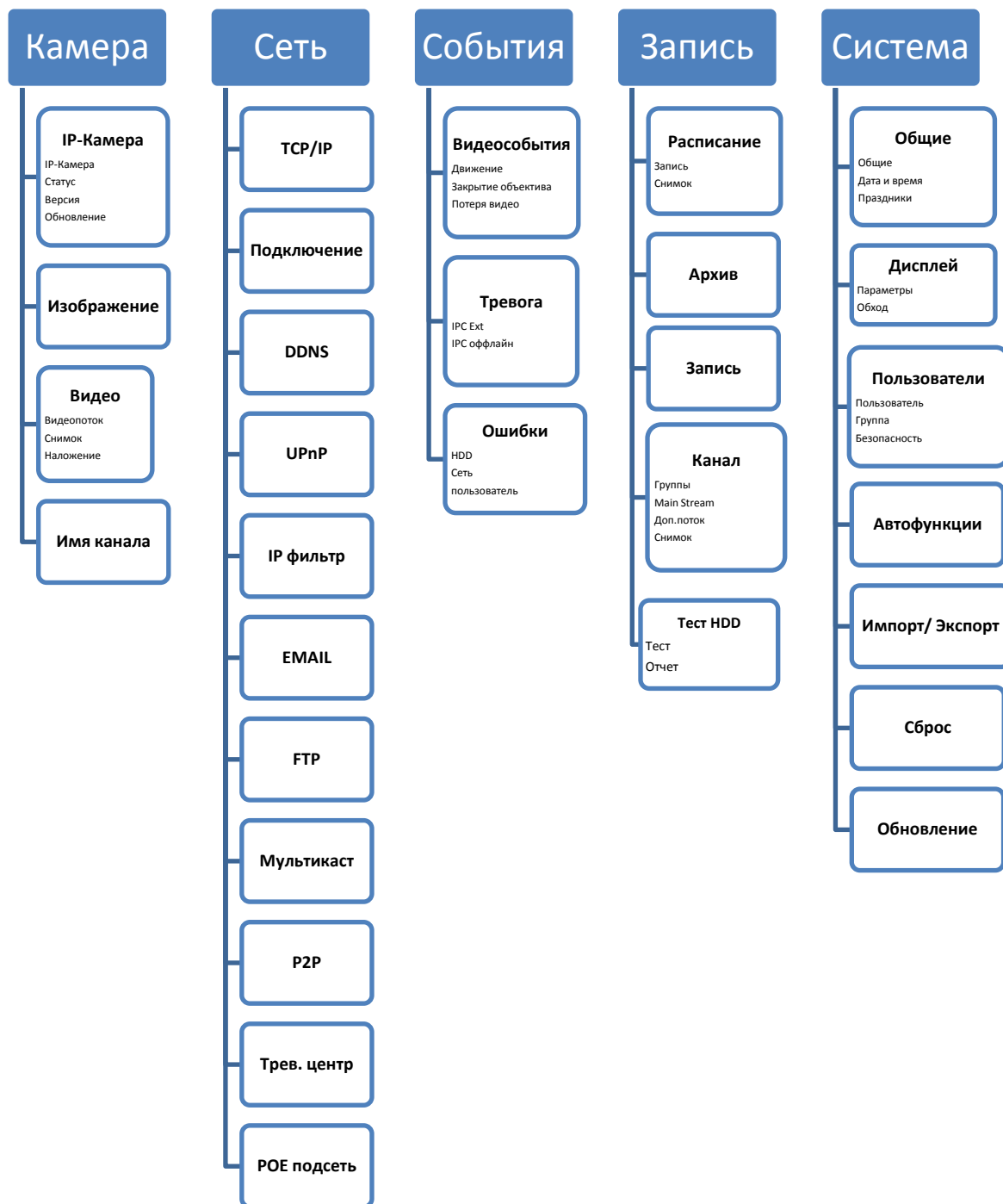
Рисунок 8.29 Схема меню «Настройка».
