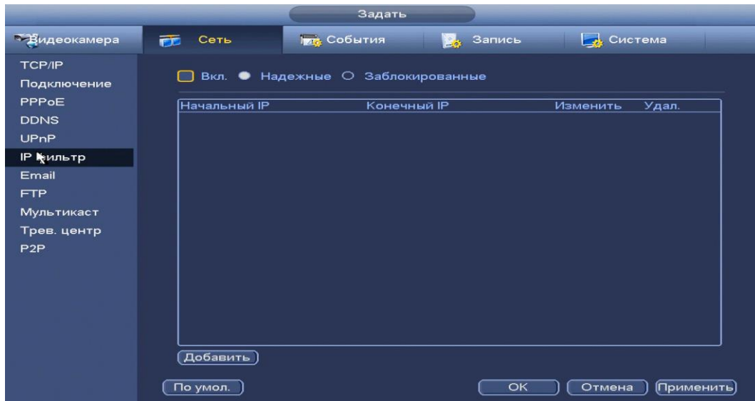
Рисунок 8.48 Интерфейс настройки «IP фильтр»
