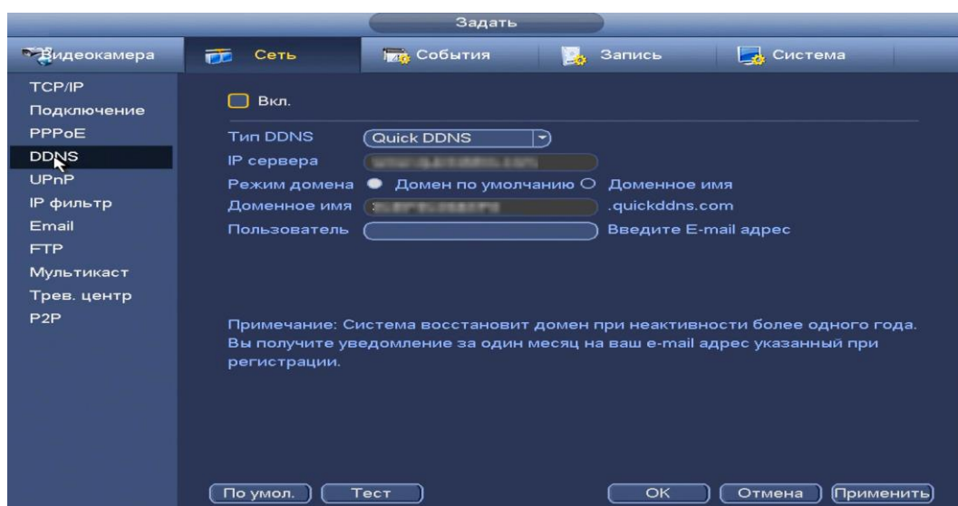
Рисунок 8.46 Интерфейс настройки «DDNS».
