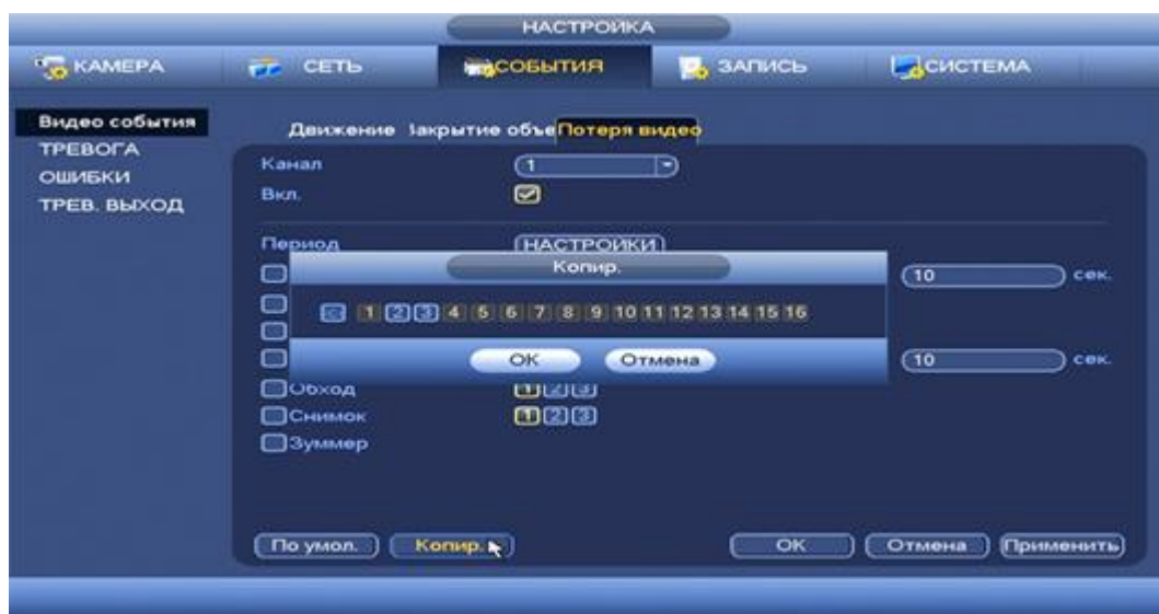
Рисунок 8.73 Копирование настроек на другие каналы.
