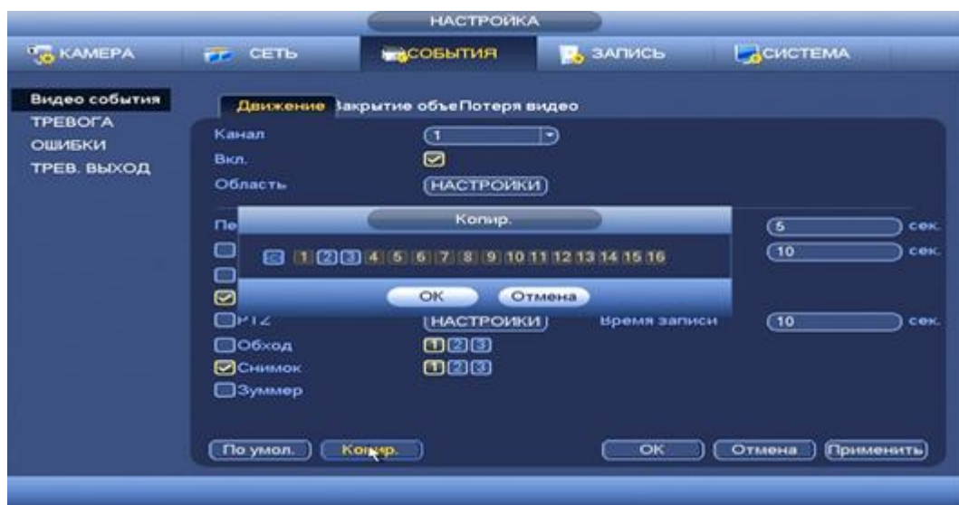
Рисунок 8.61 Копирование настроек на другие каналы.
