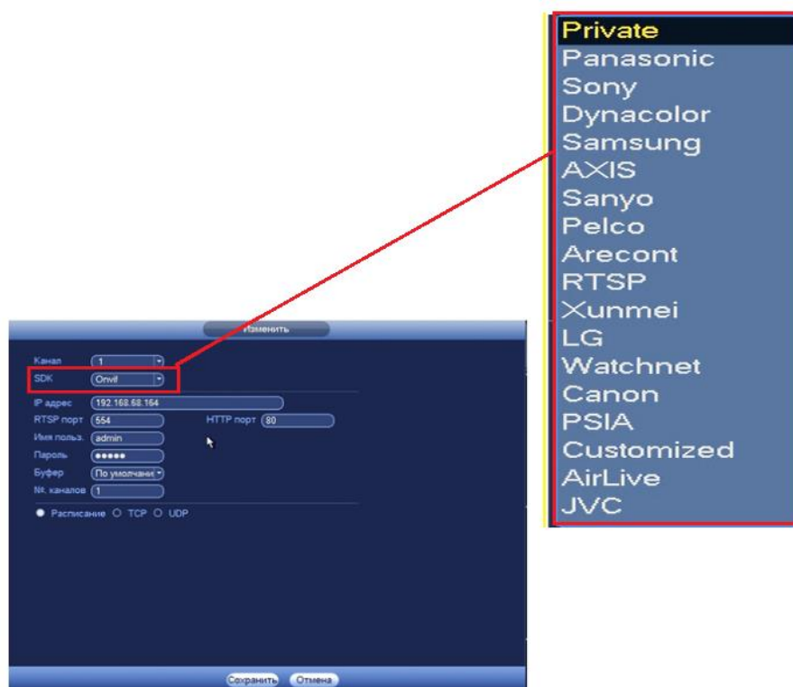
Рисунок 6.12 Настройка добавления камер сторонних производителей.
