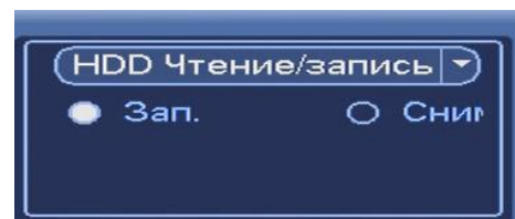
Рисунок 8.5 Тип поиска
