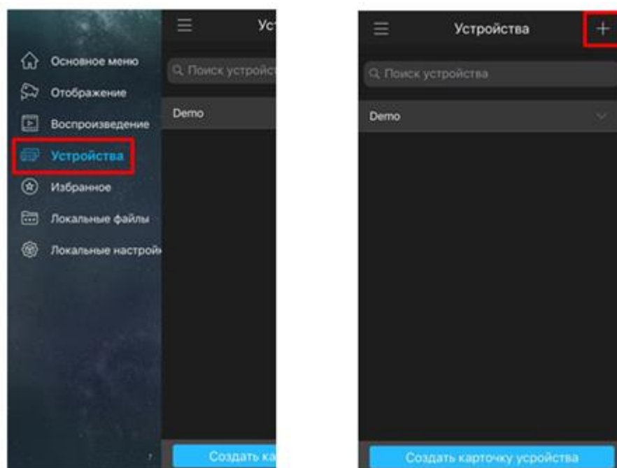
Рисунок 9.3 Меню устройства
