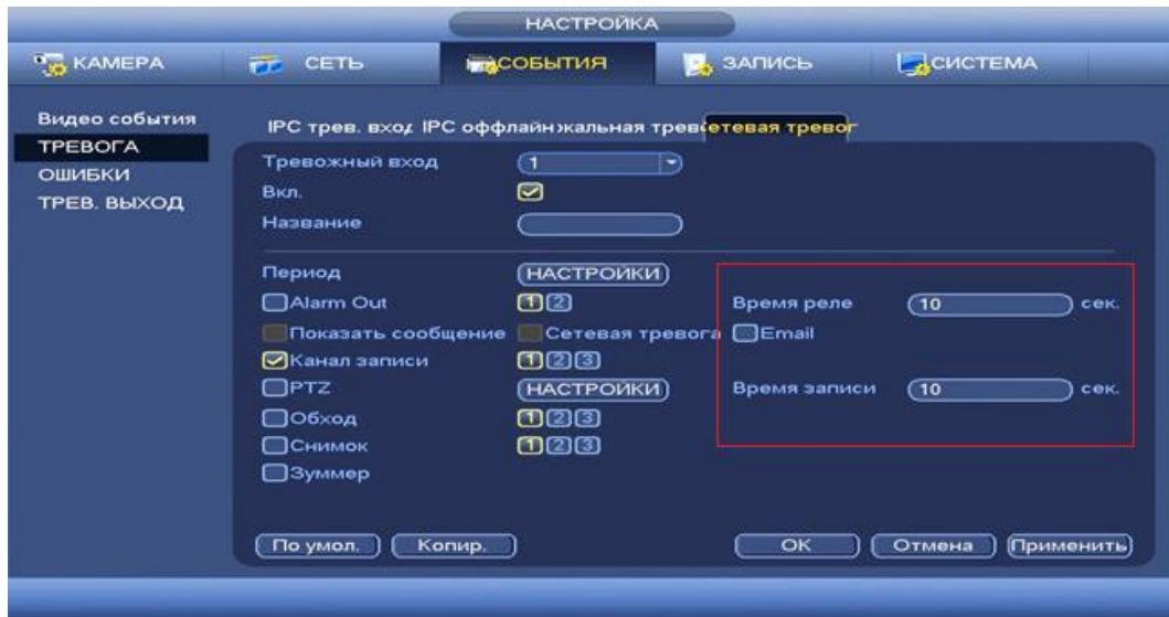
Рисунок 8.94 Установка настроек.
