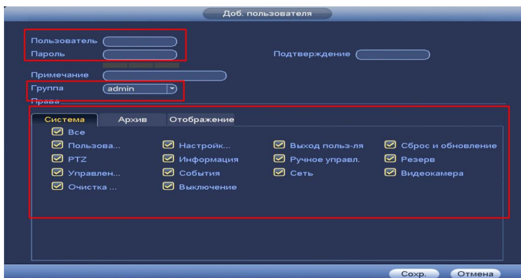
Рисунок 8.125 Назначение прав.
