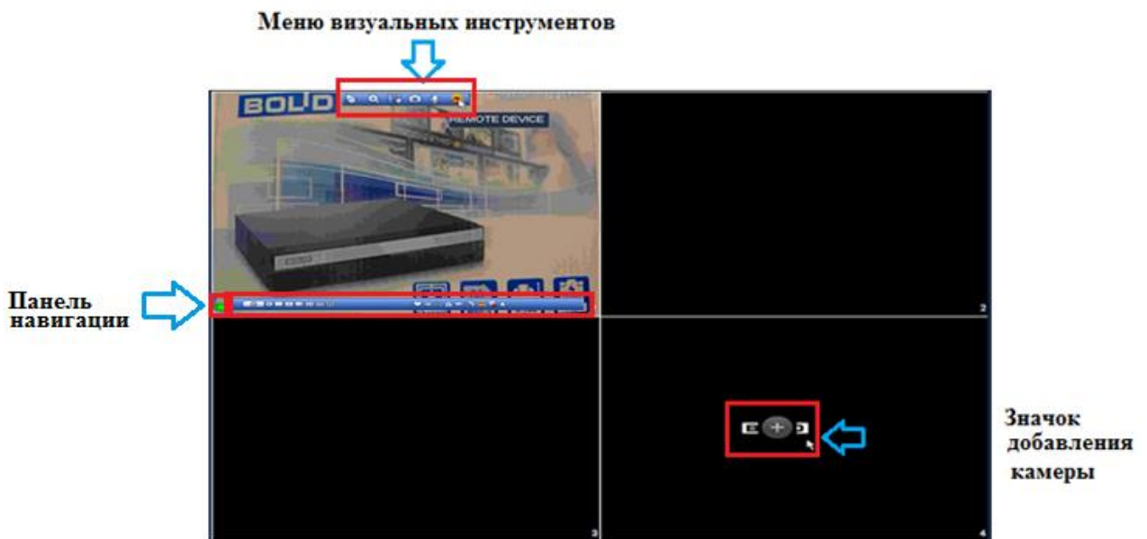
Рисунок 7.3 Добавление IP-камер.
