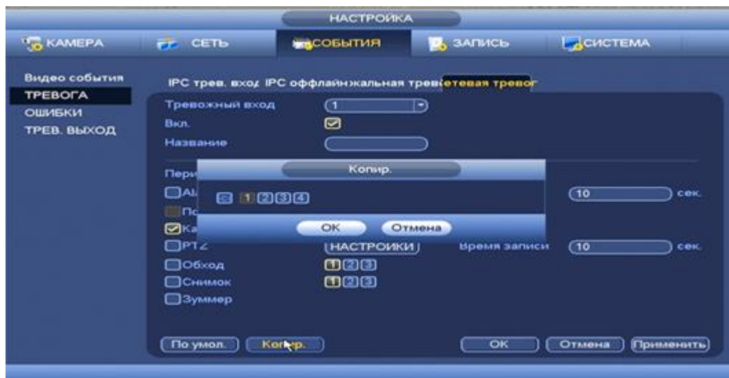
Рисунок 8.95 Копирование настроек на другие каналы.
