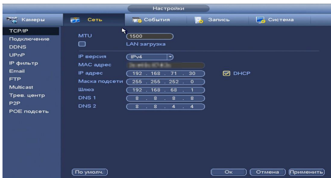
Рисунок 8.44 Интерфейс настройки «TCP/IP».
