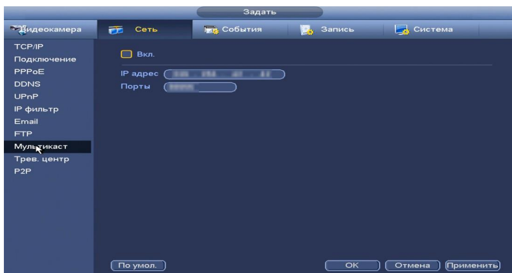
Рисунок 8.51 Интерфейс настройки «Мультикаст»
