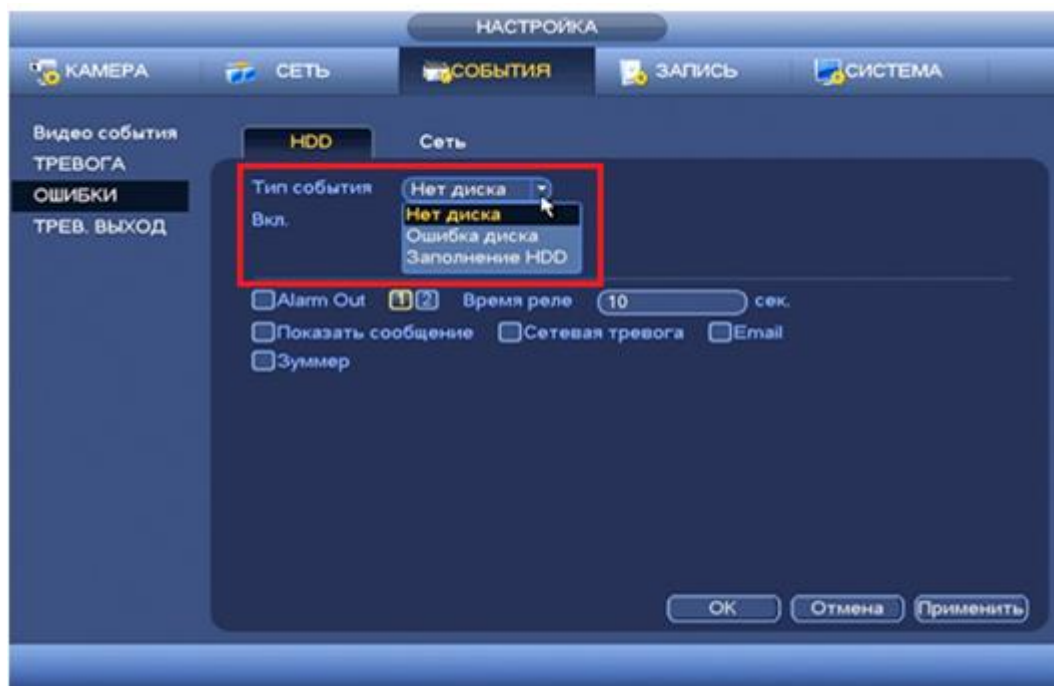
Рисунок 8.96 Интерфейс настройки HDD.
