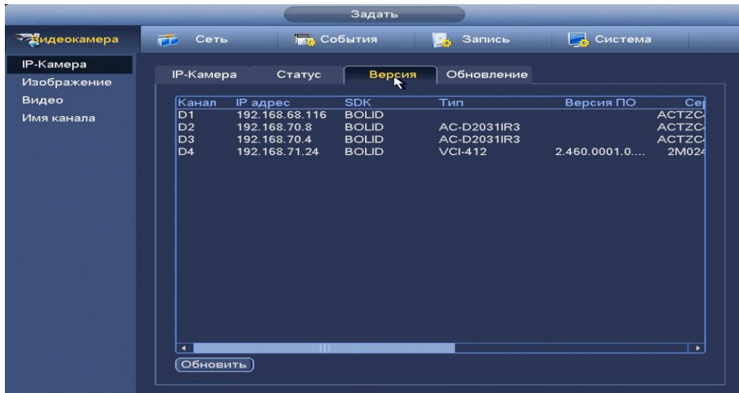
Рисунок 8.35 Интерфейс просмотра версии прошивок.
