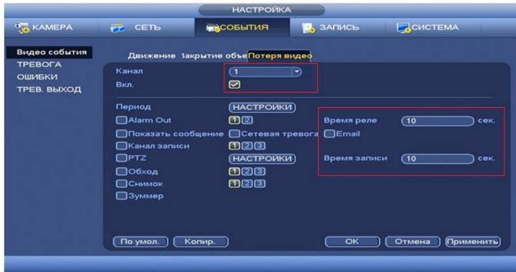
Рисунок 8.72 Установка настроек.
