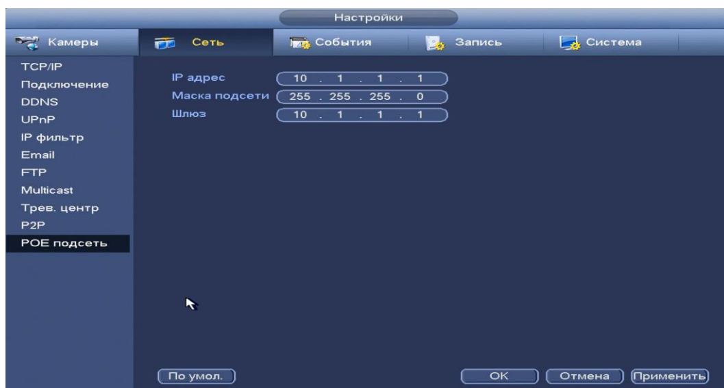
Рисунок 8.54 Интерфейс настройки.
