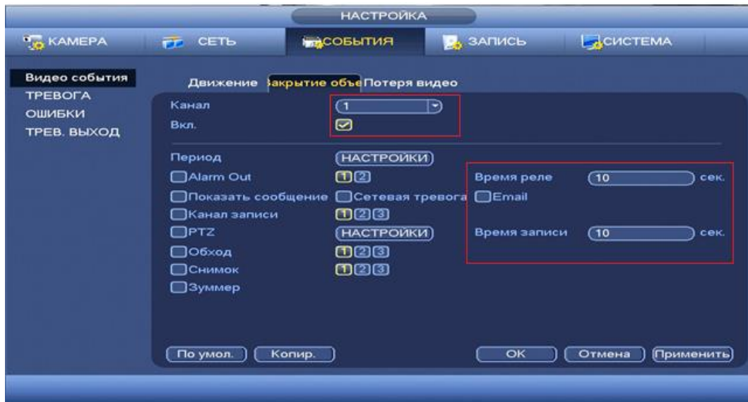
Рисунок 8.66 Установка настроек.
