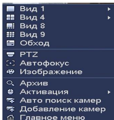
Рисунок 7.1 Контекстное меню.
