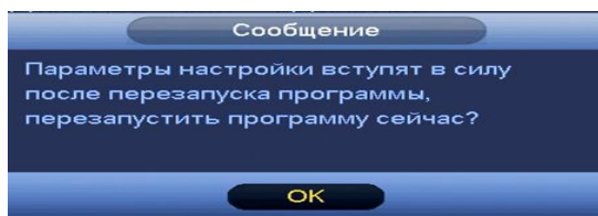
Рисунок 8.112 Всплывающее сообщение.
