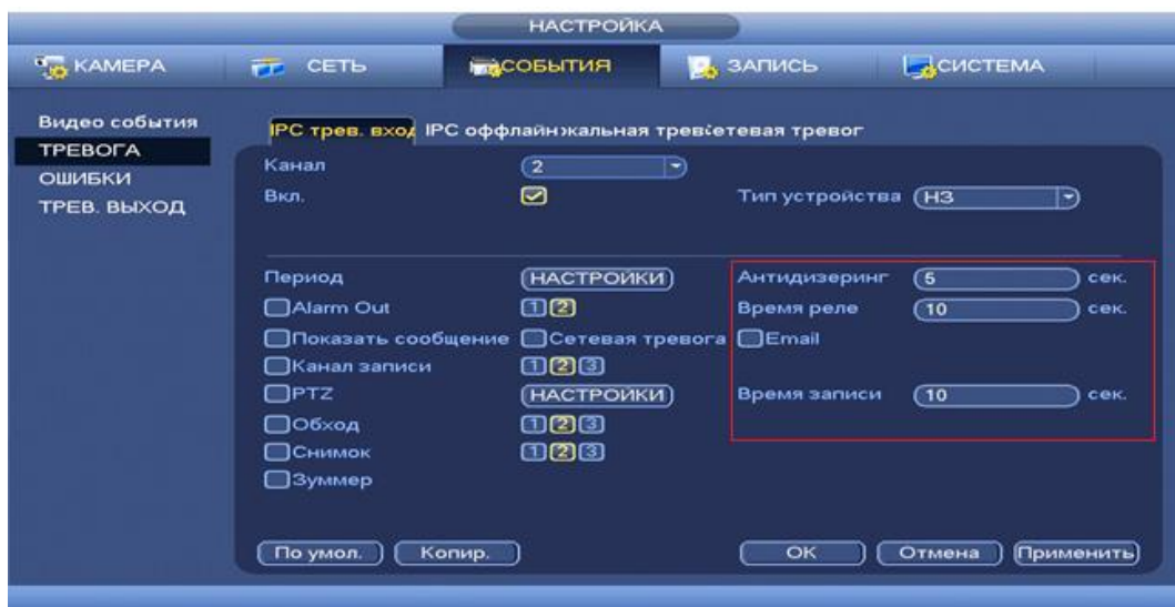
Рисунок 8.78 Установка настроек.
