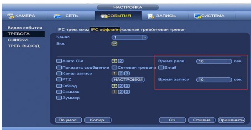
Рисунок 8.82 Установка настроек
