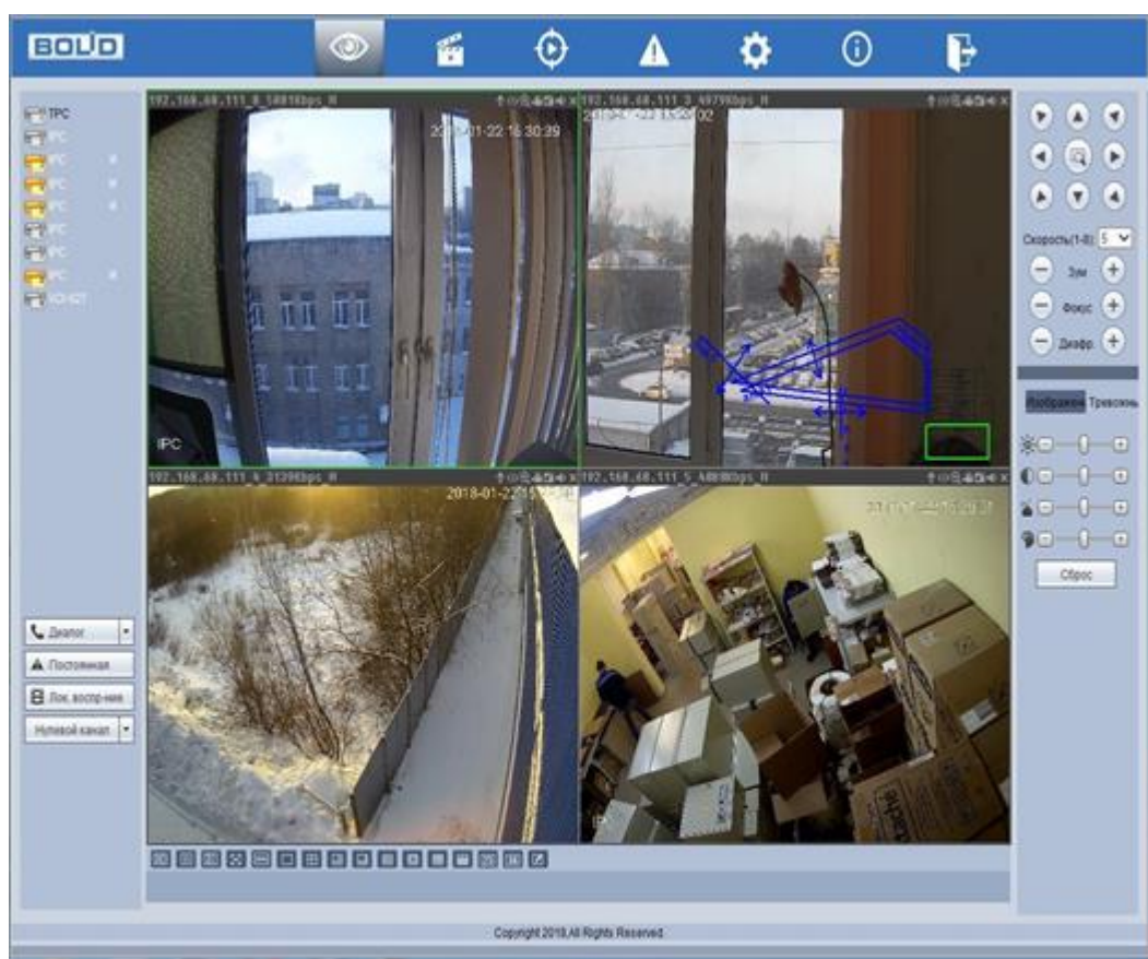
Рисунок 2.1 Web-интерфейс
