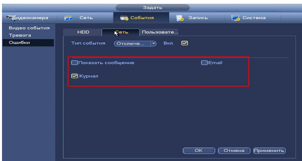
Рисунок 8.99 Установка настроек.
