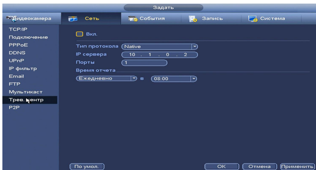
Рисунок 8.53 Интерфейс настройки «Трев. центр».
