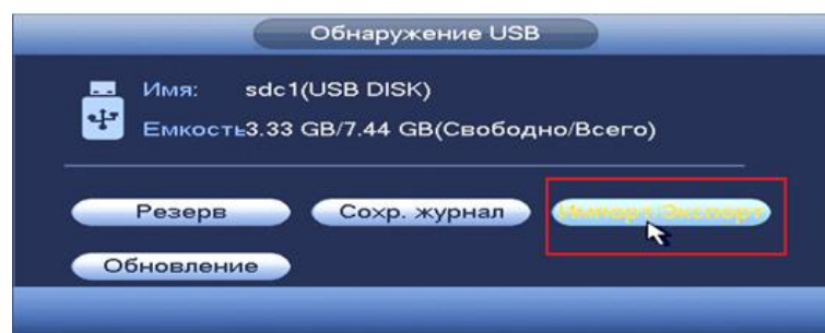
Рисунок 8.131 Всплывающее окно при подключении USB-устройства
