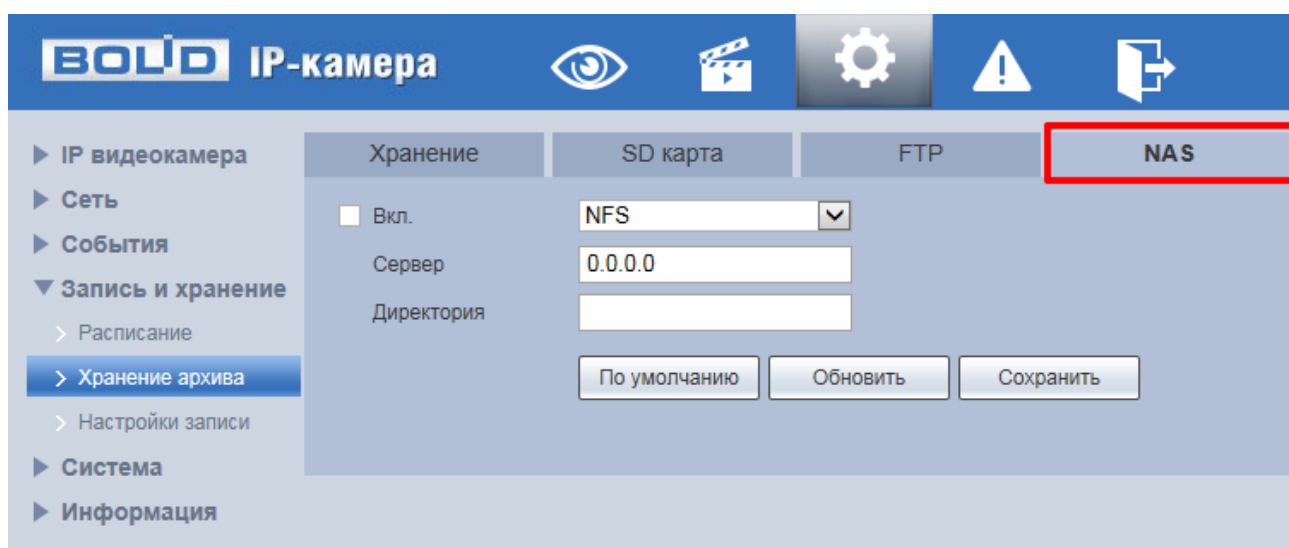
Рисунок 7.101 – Вкладка «NAS»
