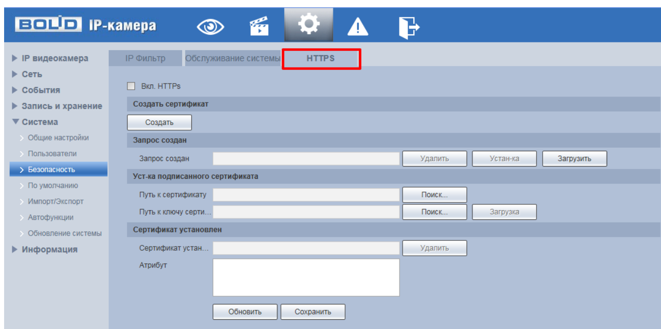
Рисунок 7.115 - Вкладка «HTTPS»
