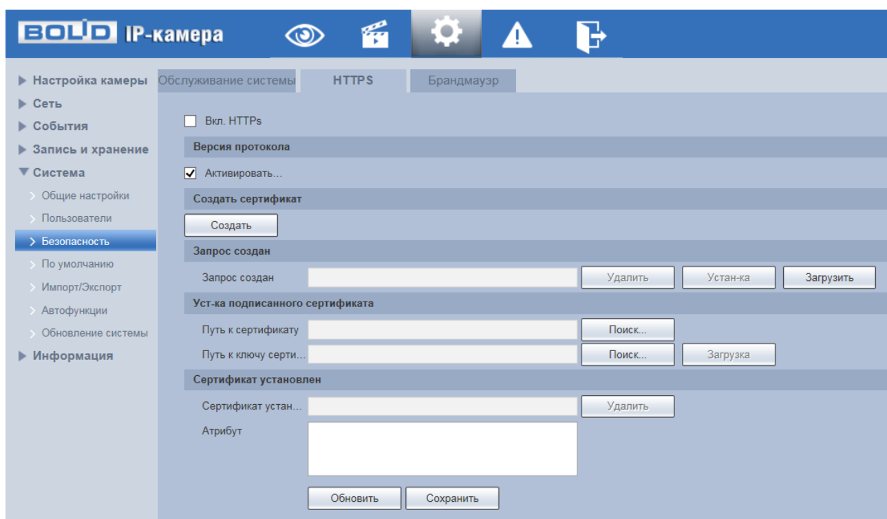
Рисунок 7.107 - Вкладка «HTTPS»
