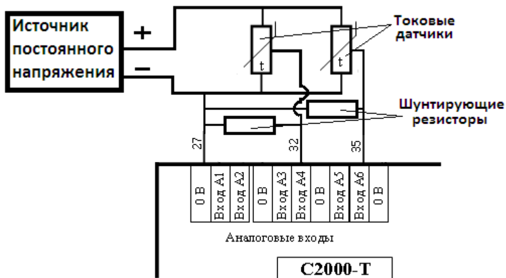
Рисунок 7. Подключение токовых датчиков
