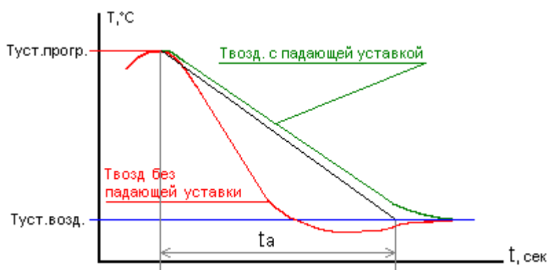
Рисунок 56. Падающая уставка
