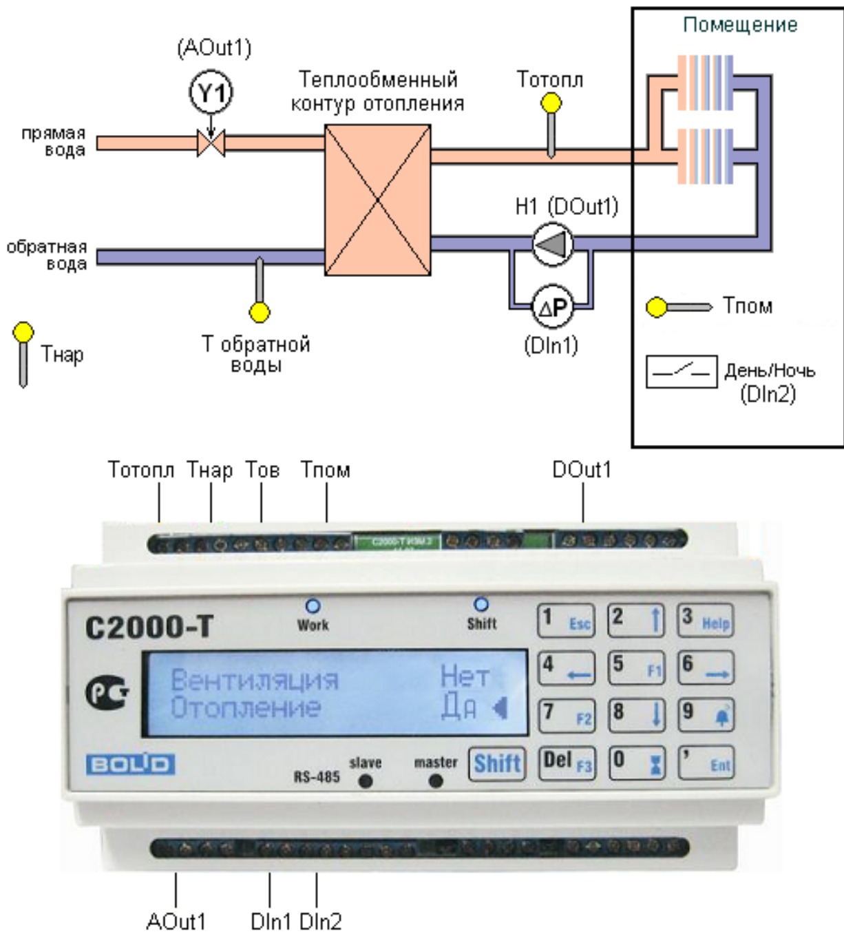
Рисунок 58. Функциональная схема системы отопления
