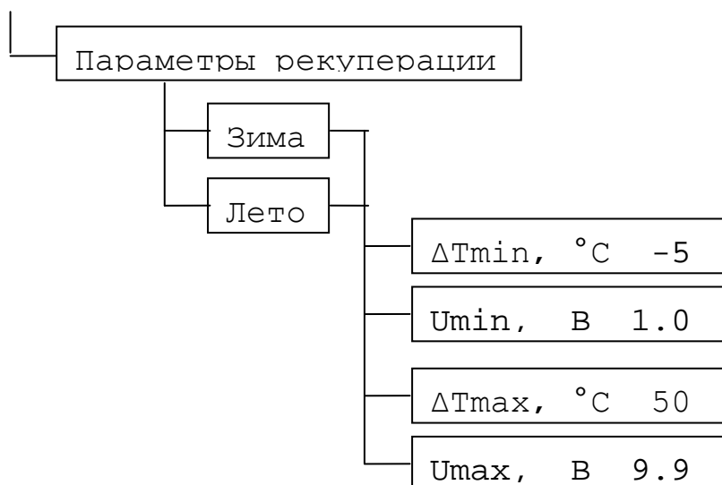
Рисунок 26. Параметры рекуперации
