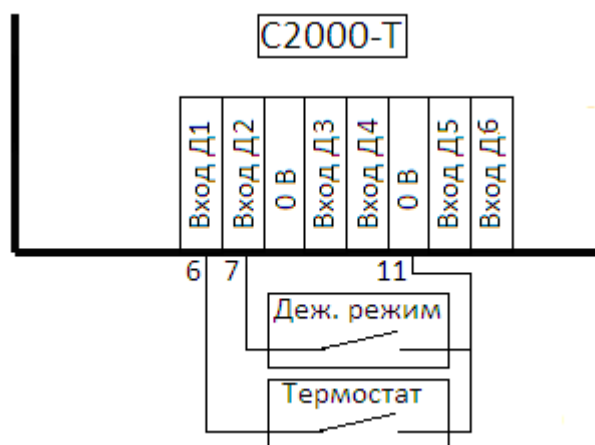
Рисунок 8. Подключение дискретных датчиков
