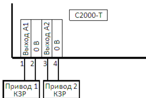
Рисунок 9. Подключение аналоговых ИМ
