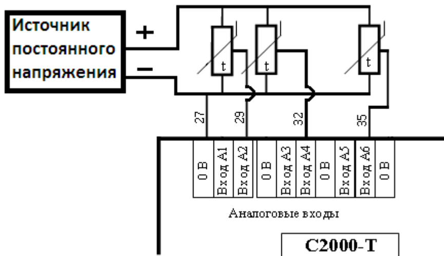
Рисунок 6. Подключение датчиков с сигналом в виде напряжения
