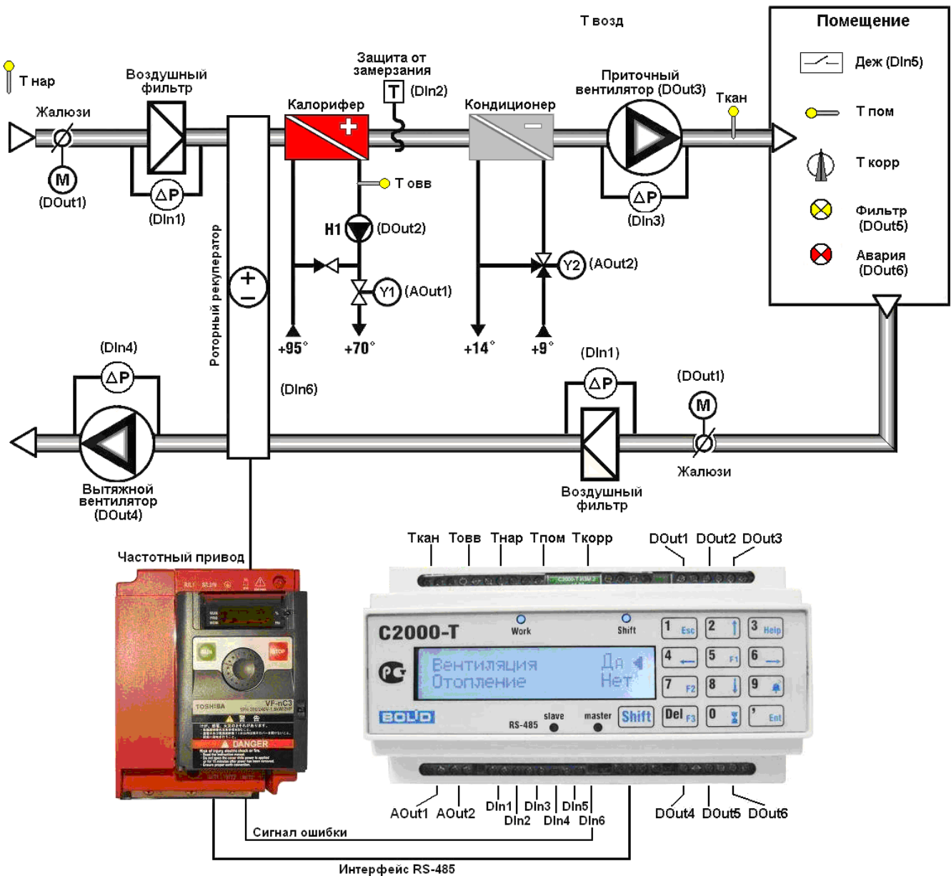
Рисунок 55. Функциональная схема системы вентиляции
