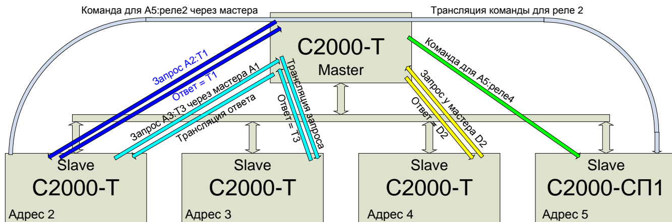
Рисунок 11. Подключение ведомых приборов
