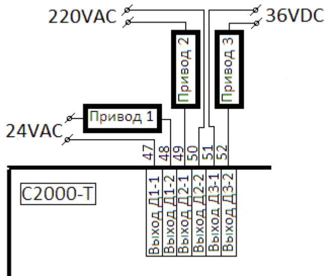
Рисунок 10. Подключение ИМ к дискретным выходам
