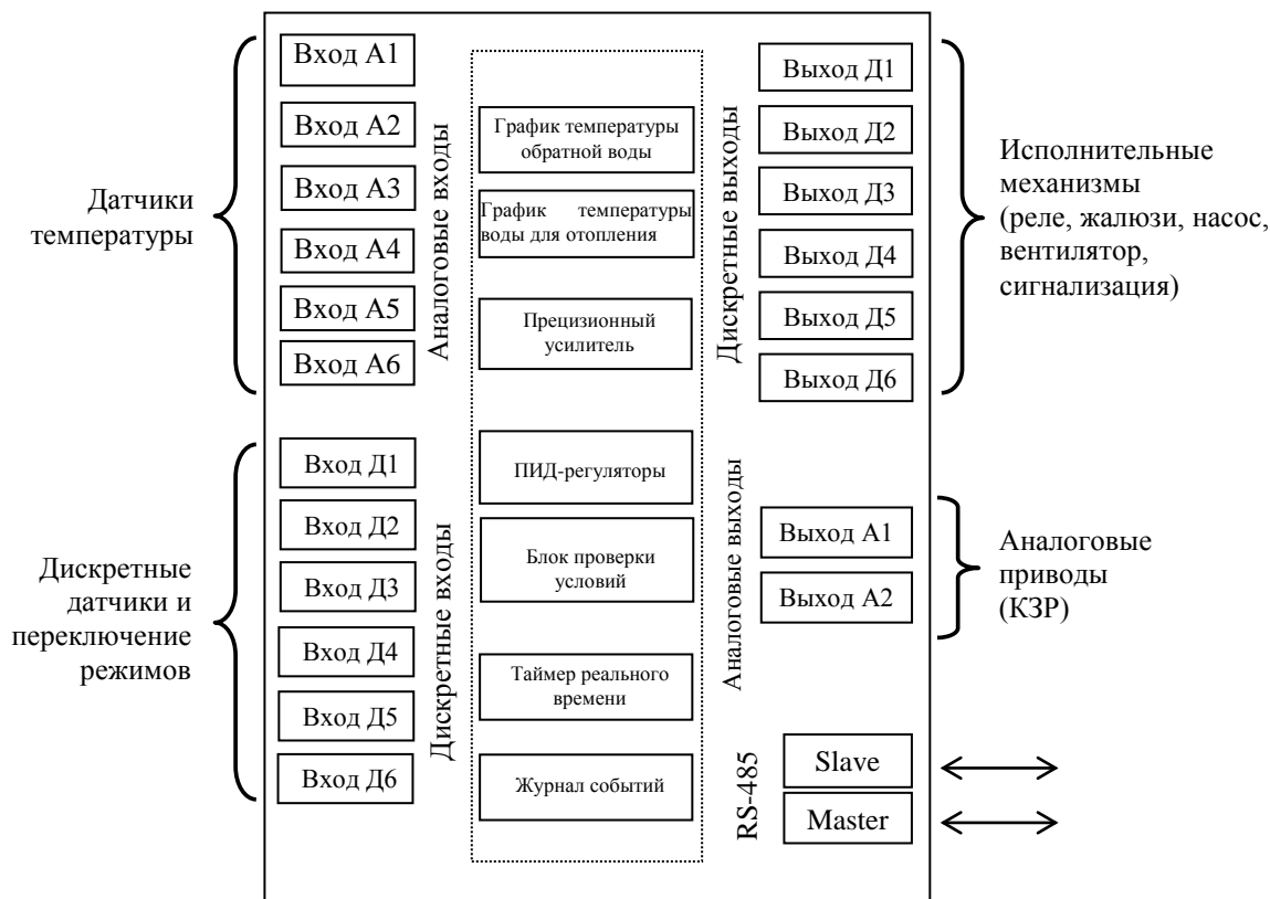
Рисунок 2. Структурная схема
