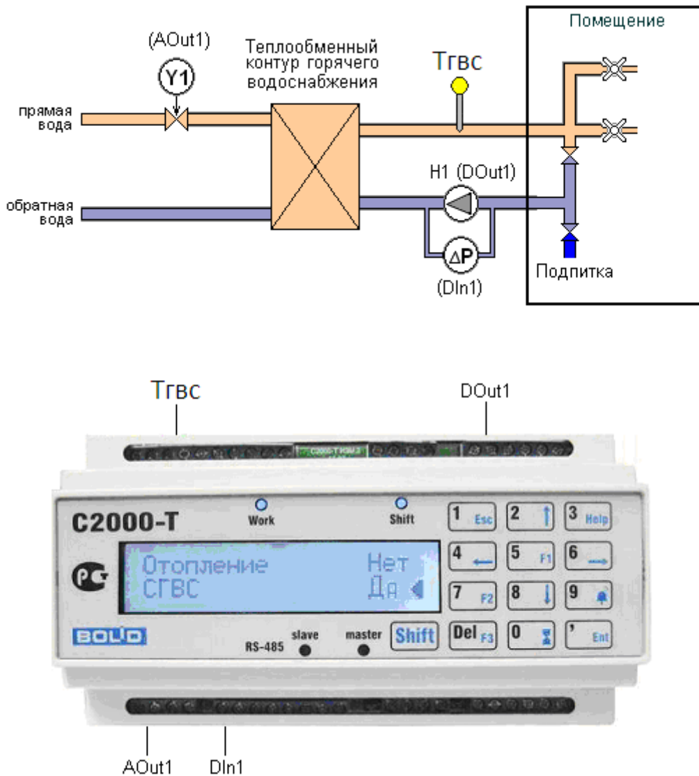
Рисунок 60. Функциональная схема системы горячего водоснабжения
