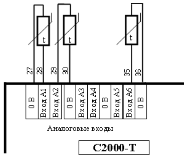
Рисунок 4. Подключение ТС по двухпроводной схеме
