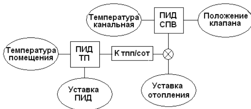
Рисунок 59. Каскадное регулирование в СОТ
