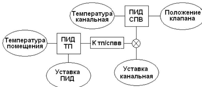
Рисунок 57. Каскадное регулирование в СПВ
