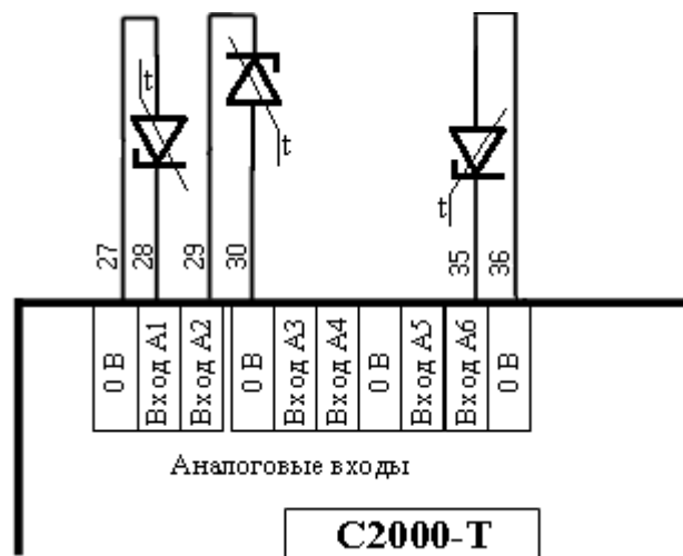
Рисунок 5. Подключение датчиков LM235
