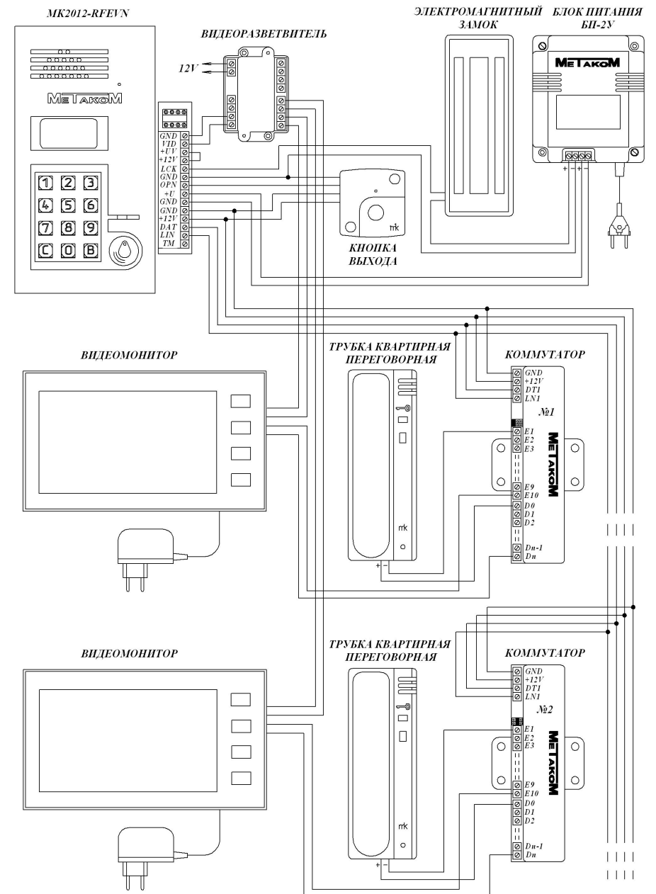
Рис. 2 Пример монтажа блока вызова MK2012-RFEVN
