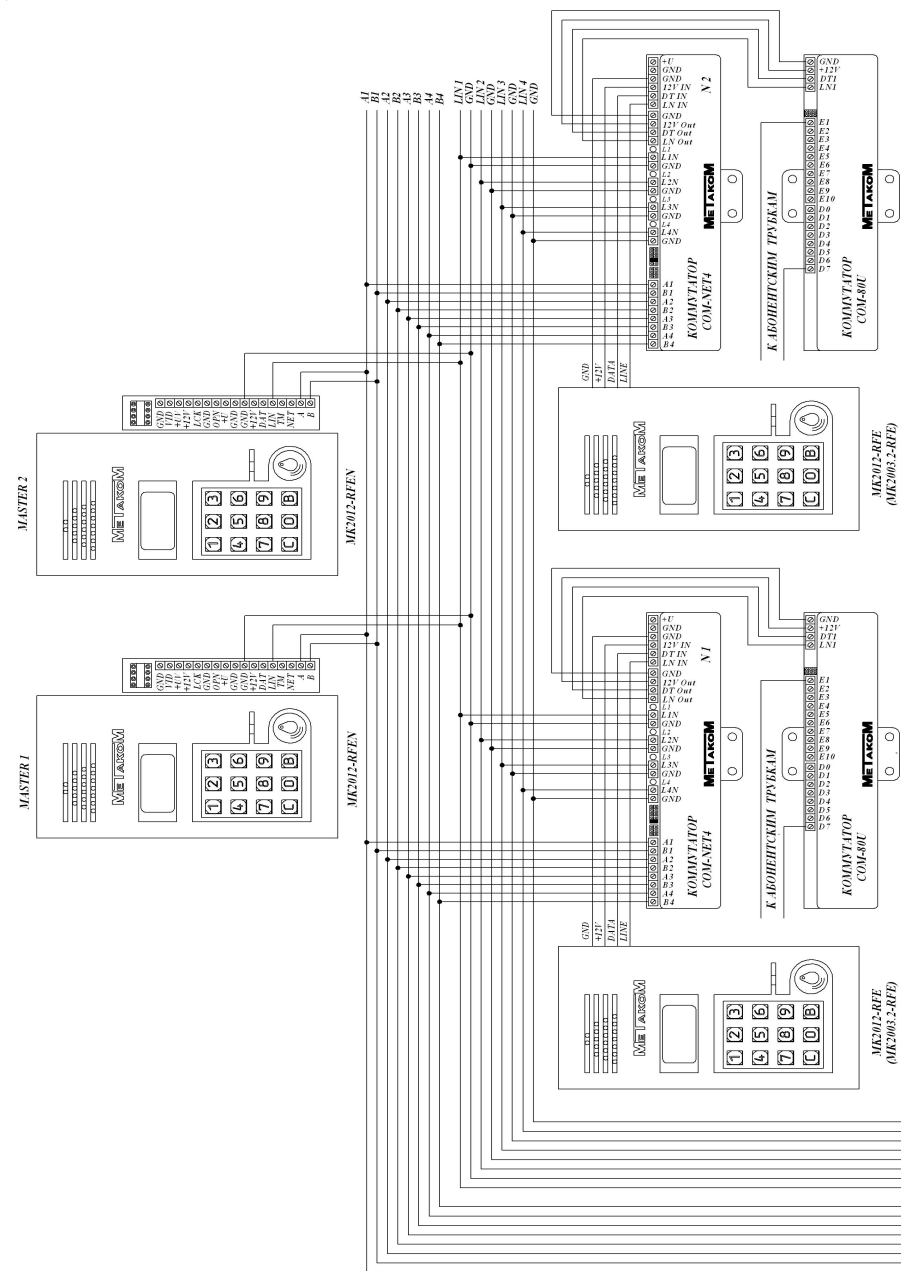
Рис. 4.1 Пример монтажа блока вызова MK2012-RFEN для огороженных территорий с несколькими входами на территорию с использованием сетевых коммутаторов.
