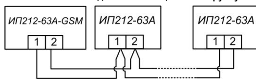
Рис.5 Схема соединения извещателей в группу
