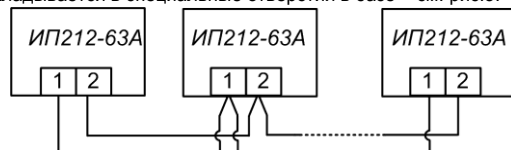
Рис.4 Схема соединения извещателей в группу
