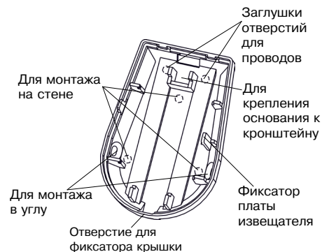
Рисунок 2 – Основание
