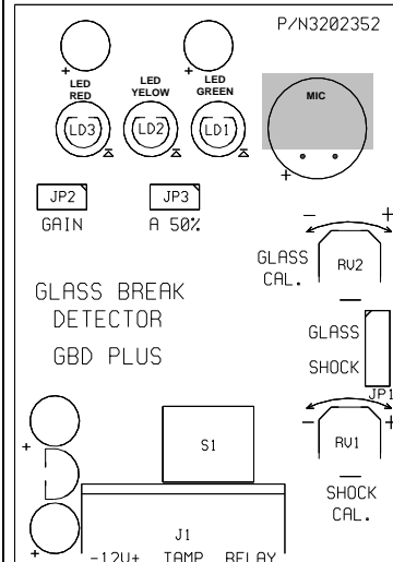
Рис. 4 - ПЕЧАТНАЯ ПЛАТА
