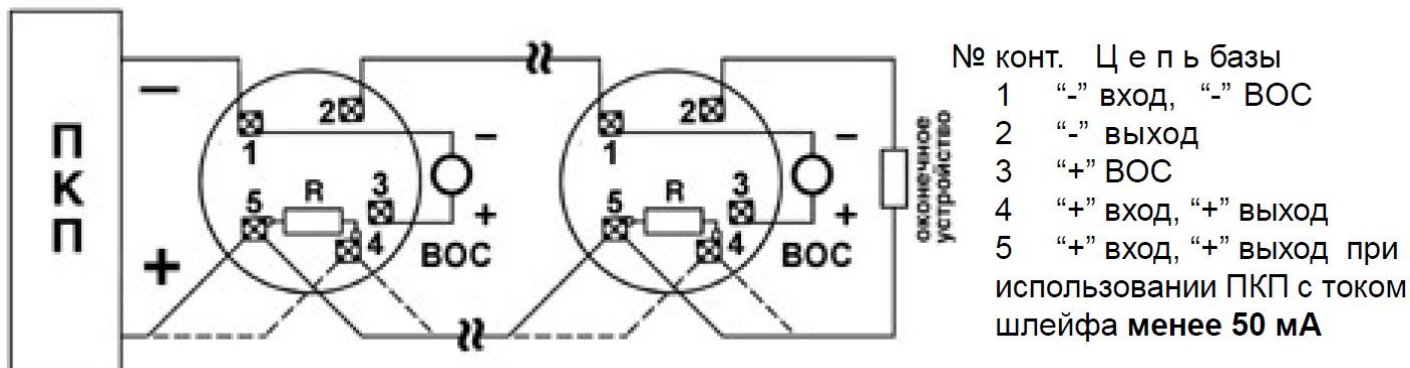
Рис.1. Схема подключения извещателей ИП212-58М с базами E1000R, E1000B к ПКП.
