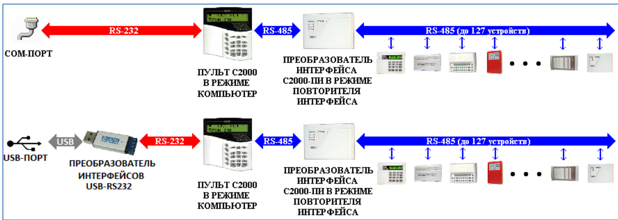
Схема подключения приборов к одному COM-порту/USB-порту компьютера по протоколу «Орион Про» (с гальванической развязкой).
