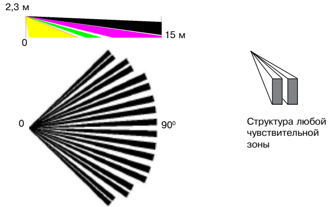
Рисунок 1 - Диаграмма зоны обнаружения
