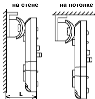
Рисунок 2 - Основание извещателя и кронштейн
