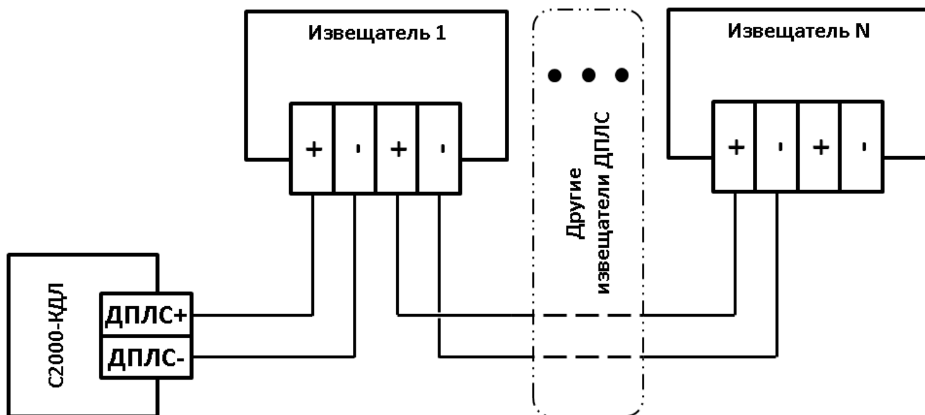
Схема подключения извещателя к контроллеру «С2000-КДЛ»
