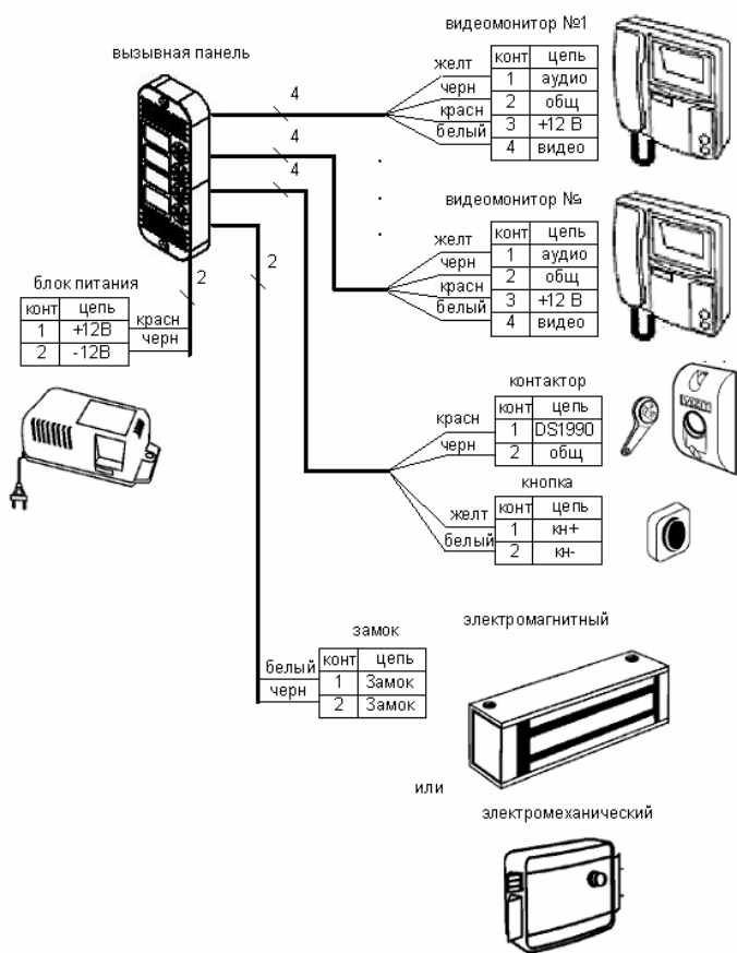
Рисунок 3.1 Схема подключения вызывной панели
