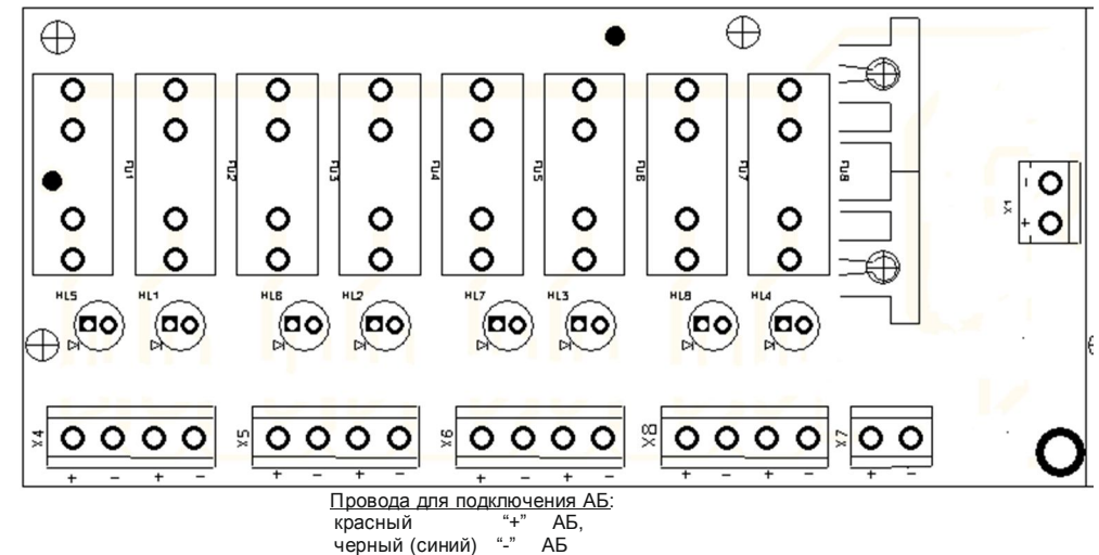
Рис. 1. Схема подключения УЗК-8Р
